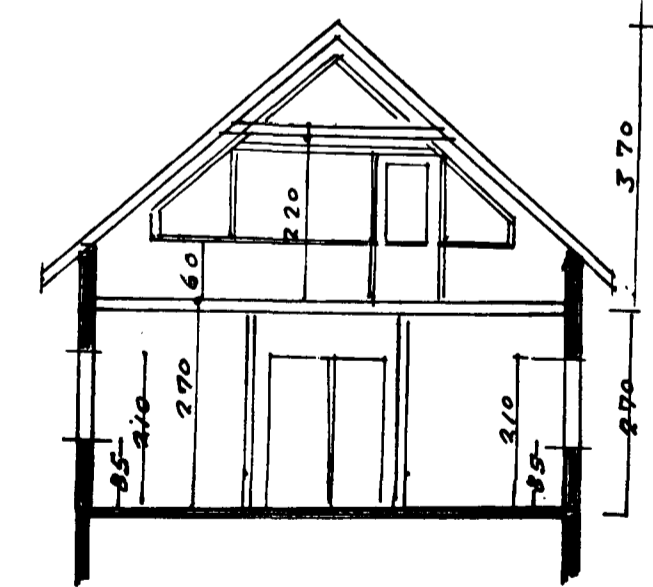
SKURÐUR AA
