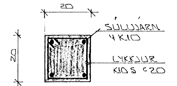
SÚLA S1 • 1:10
