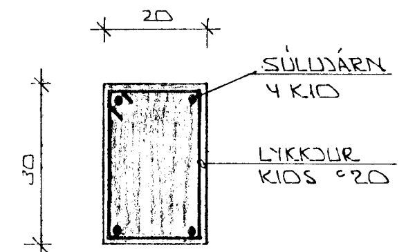
SÚLA S2 • 1:10
