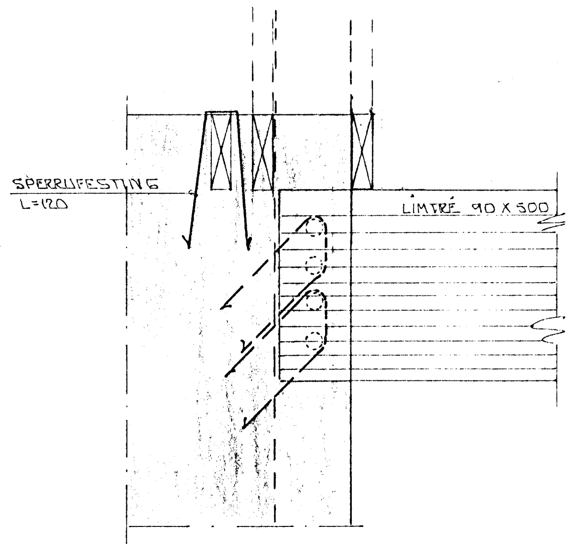
ÁSYNÐ X - X 1:10
