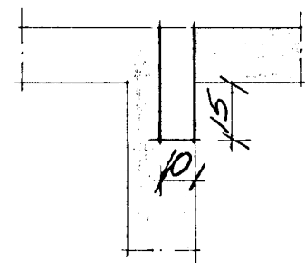
Snid A1-A1 M1:20
