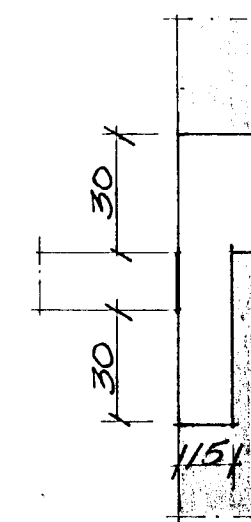
Snid A2-A2 M1:20
