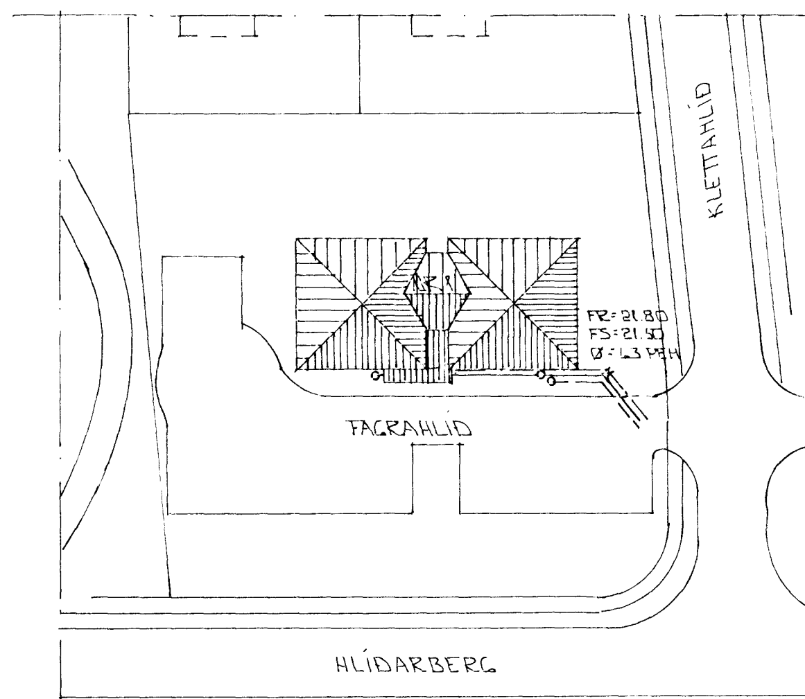
AFSTÖÐUMYND • 1 : 500
