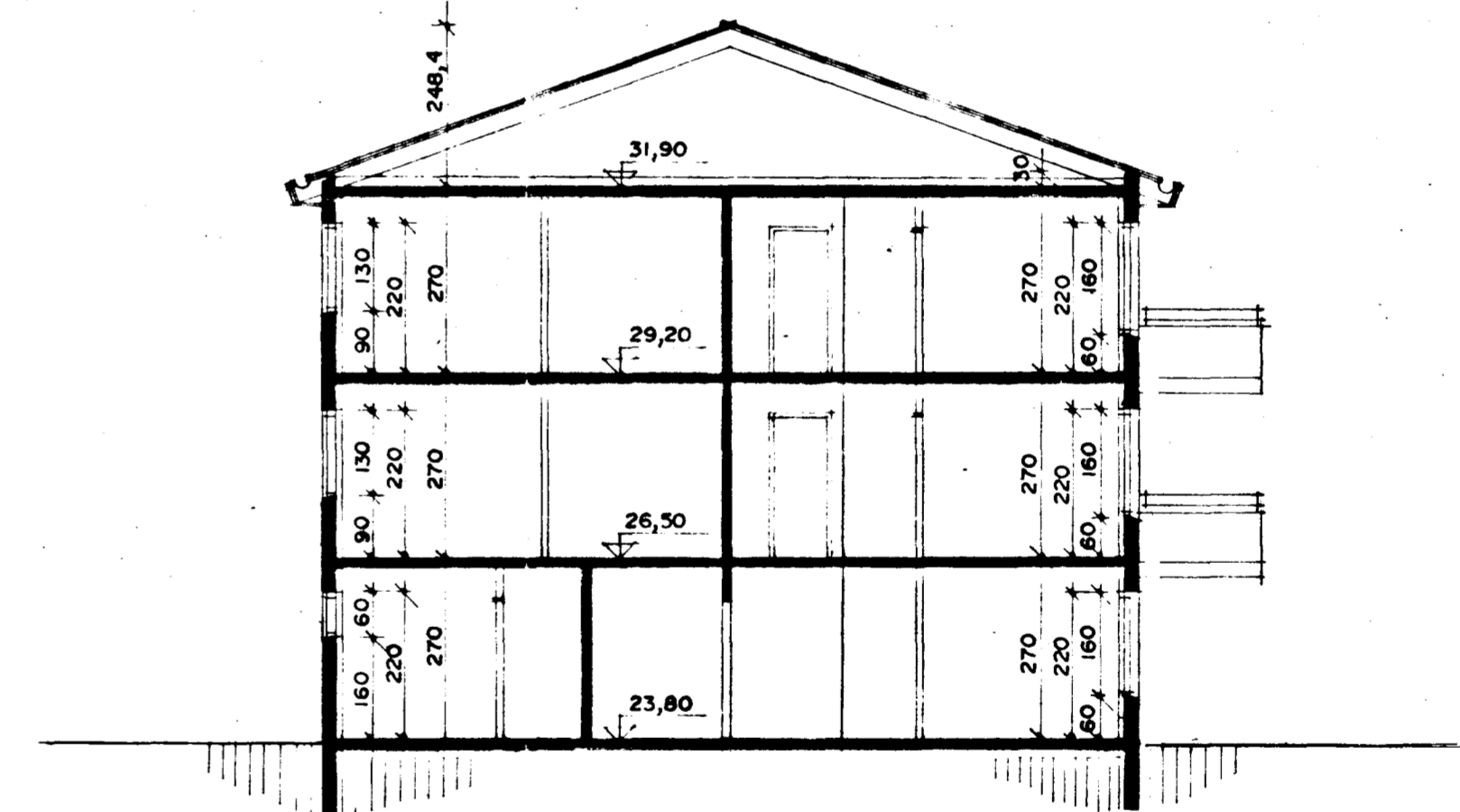
SNÐ B-B M.1:100
