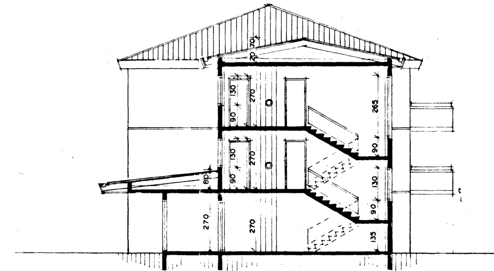
SNÐ A-A M.1:100
