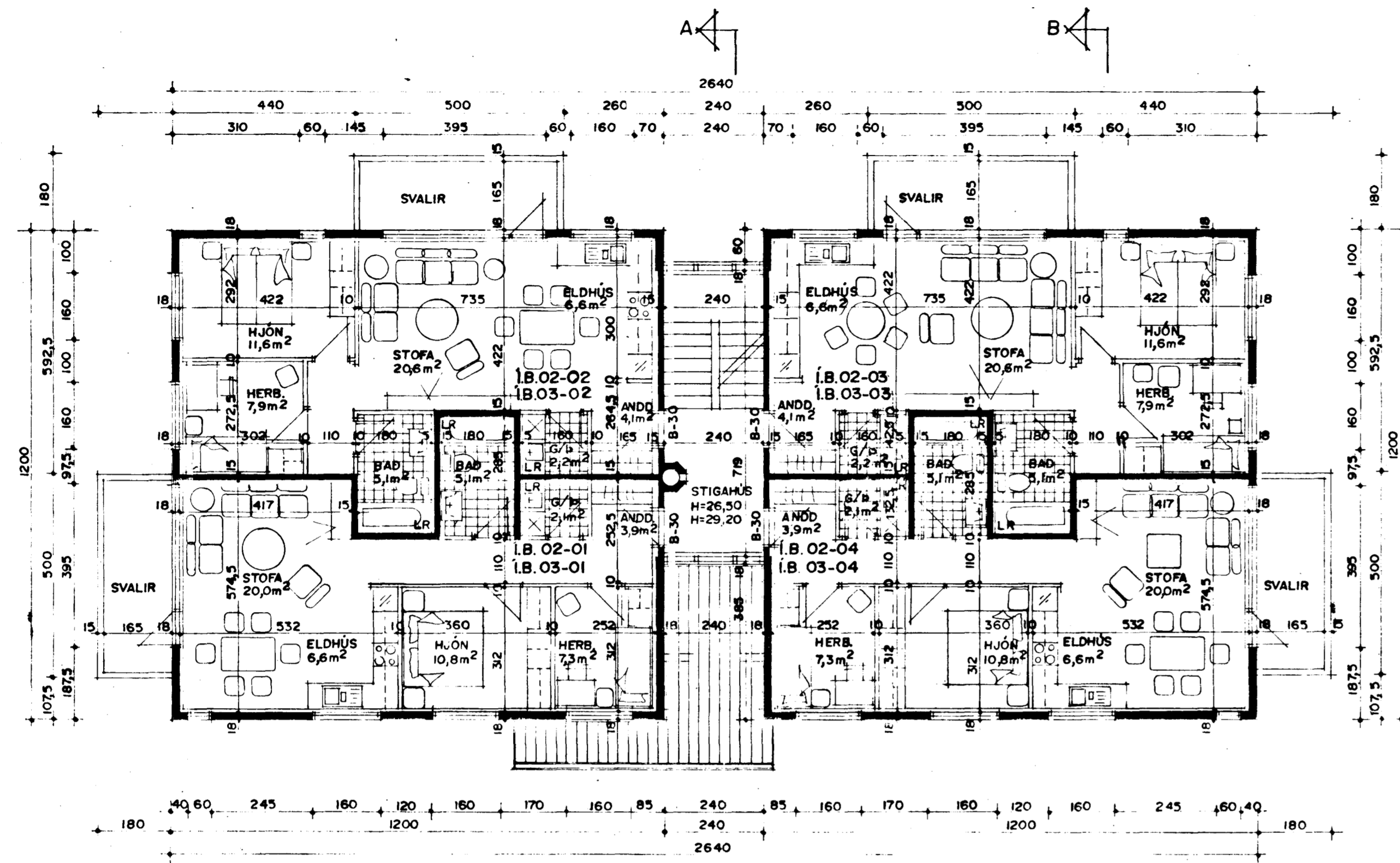
GRUNNMYND 2. OG 3. HÆÐAR M.1:100
