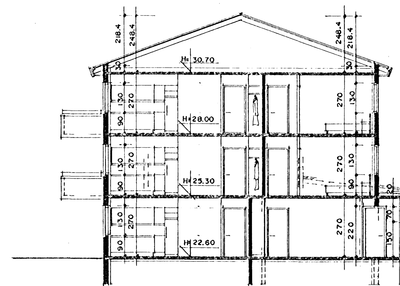
SNEIÐING A-A MKV. 1:100
