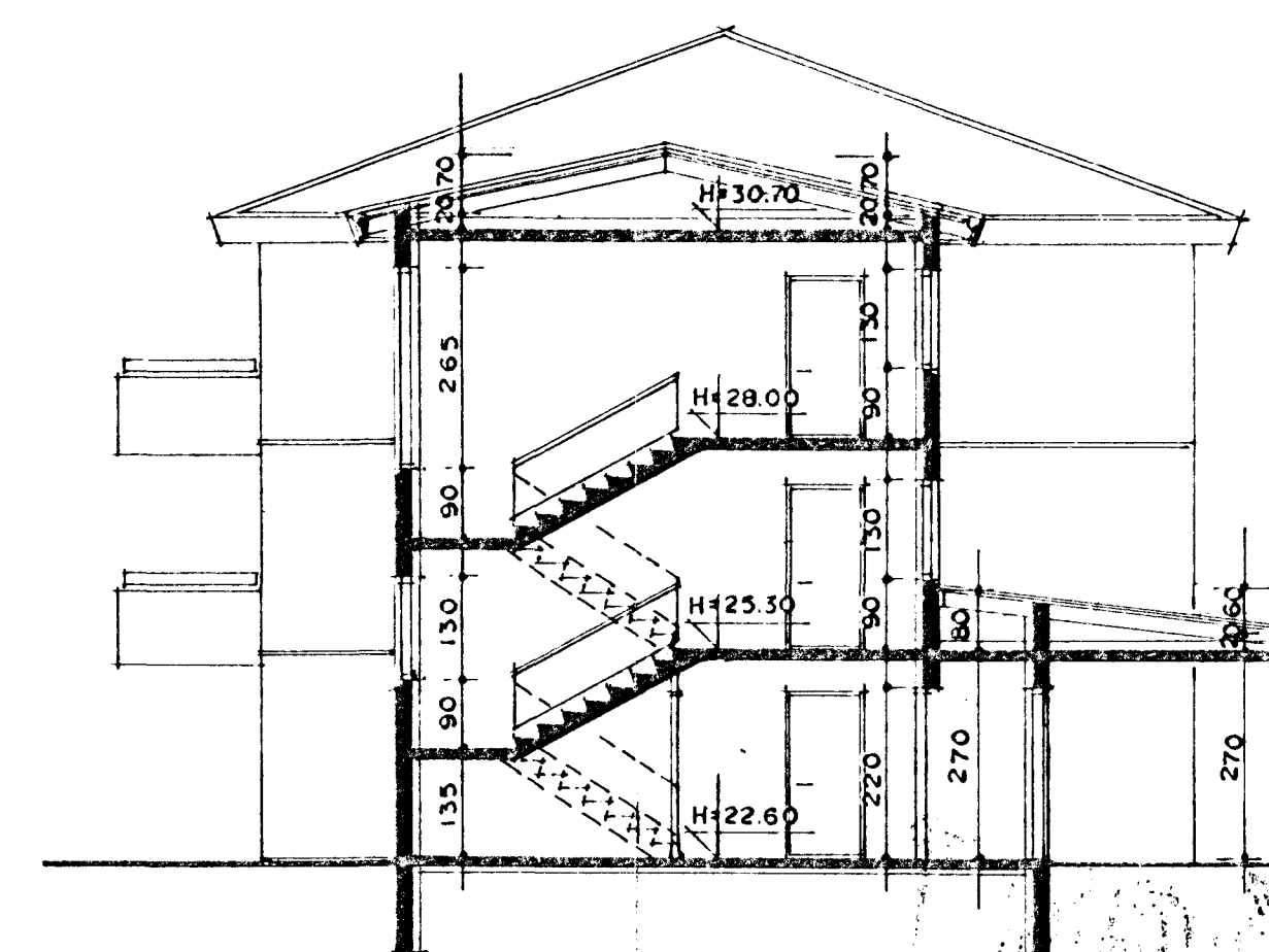
SNEIÐING B-B MKV. 1:100
