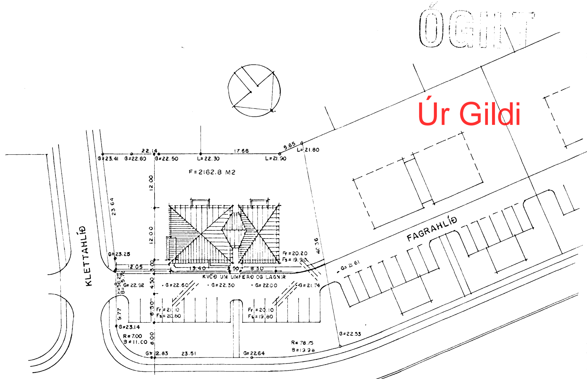
AFSTÖÐUMYND MKV. 1:500
