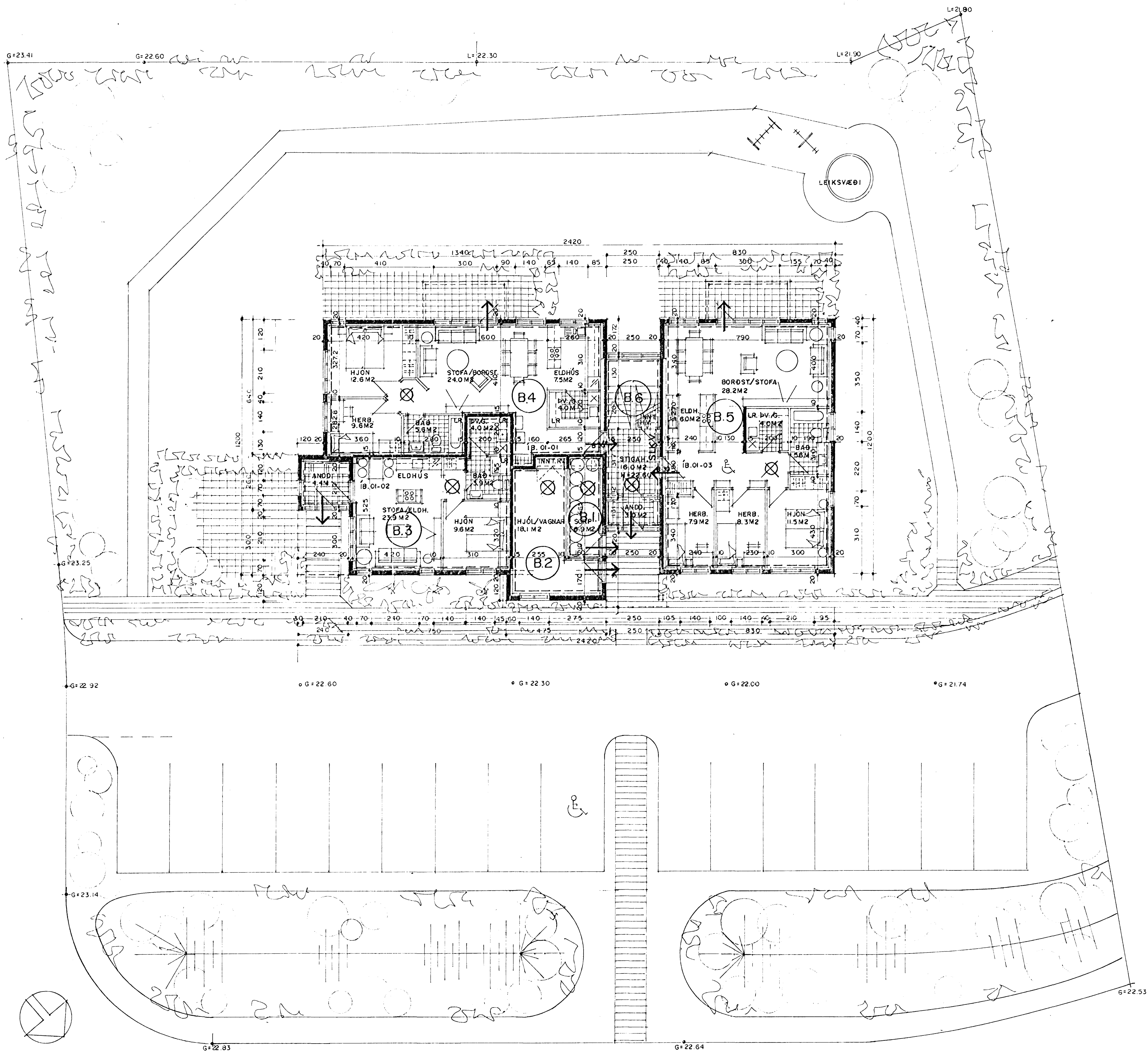
GRUNNMYND JARÐHÆÐAR MKV. 1:100
