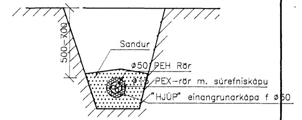
Snið A-A 1:20
