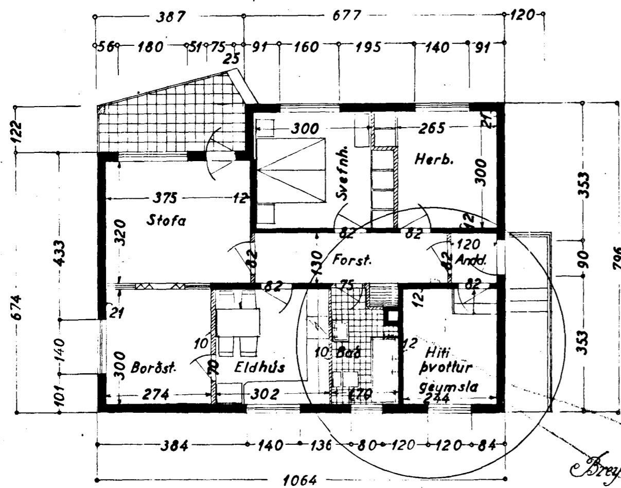
Grundmynd
