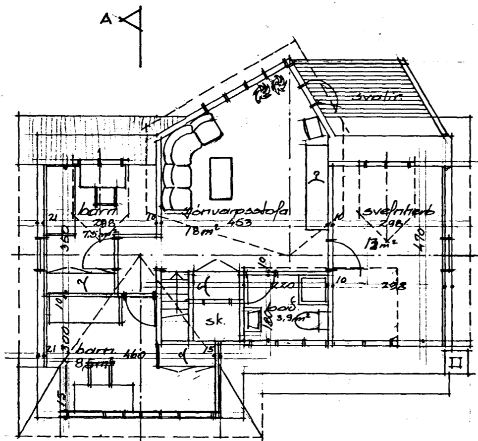
EISLHÆÐ
