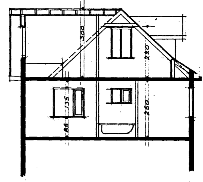
SKURÐUR A-A
