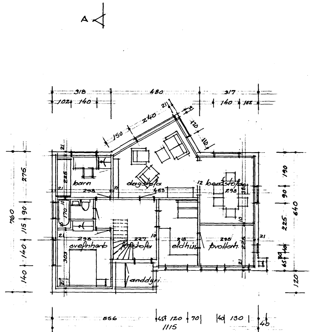
1. HÆÐ
