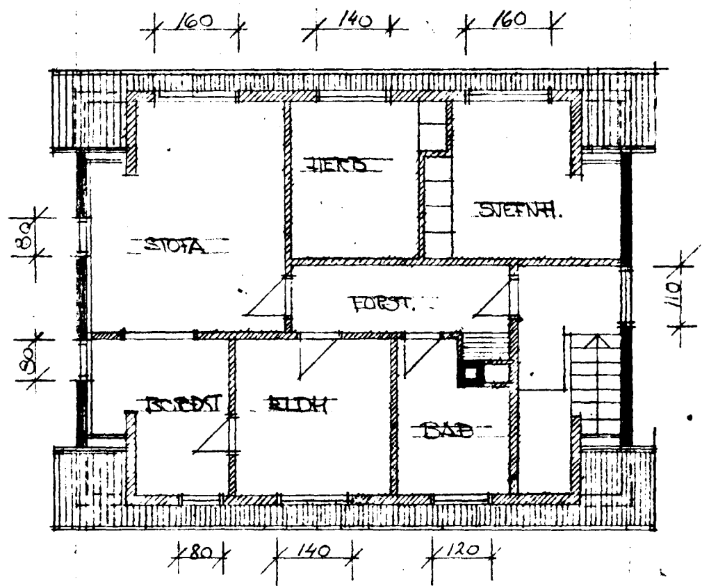
2. HÆÐ M. 1:100
