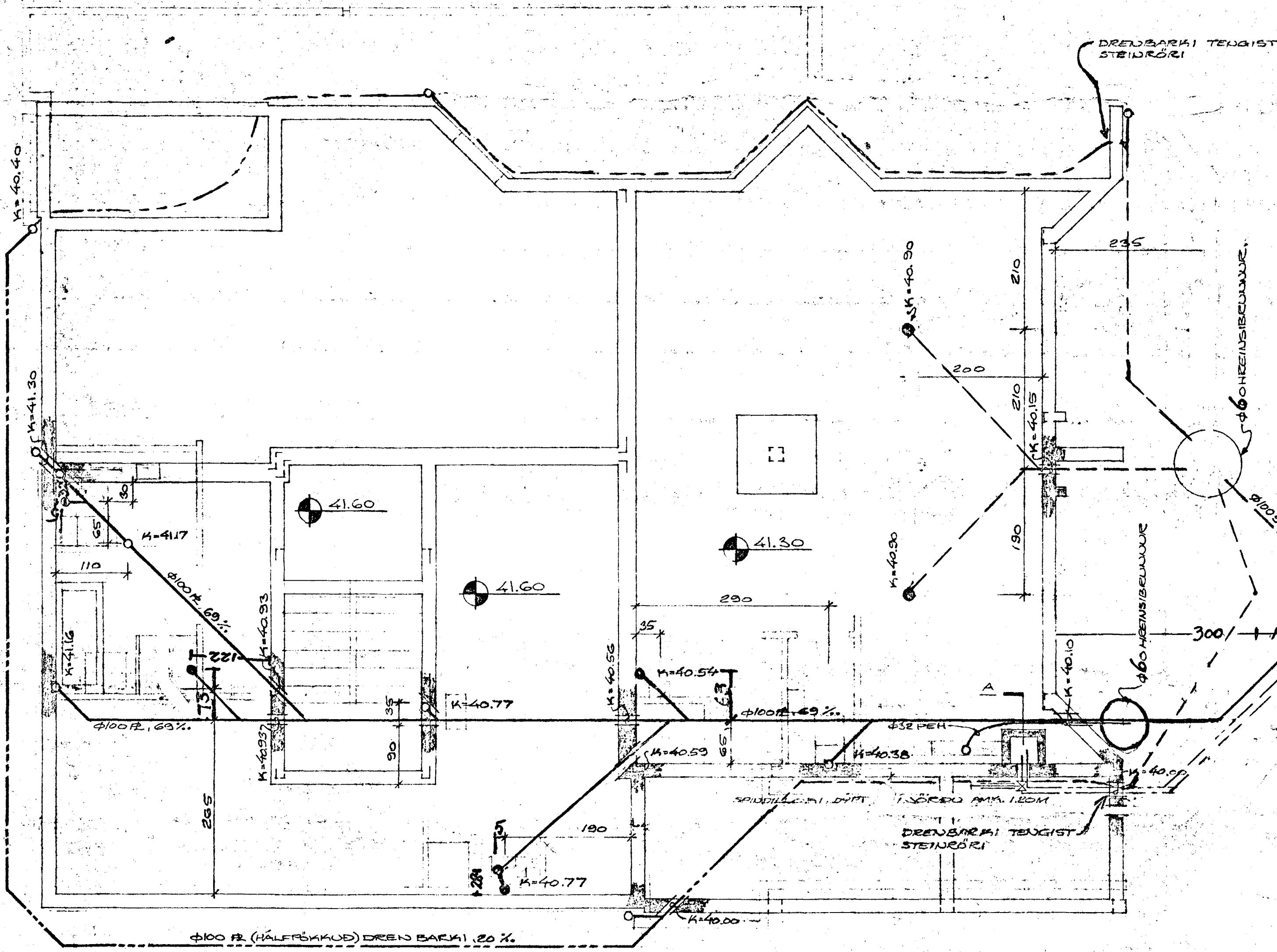
GRUNNMÝND M=1:50
