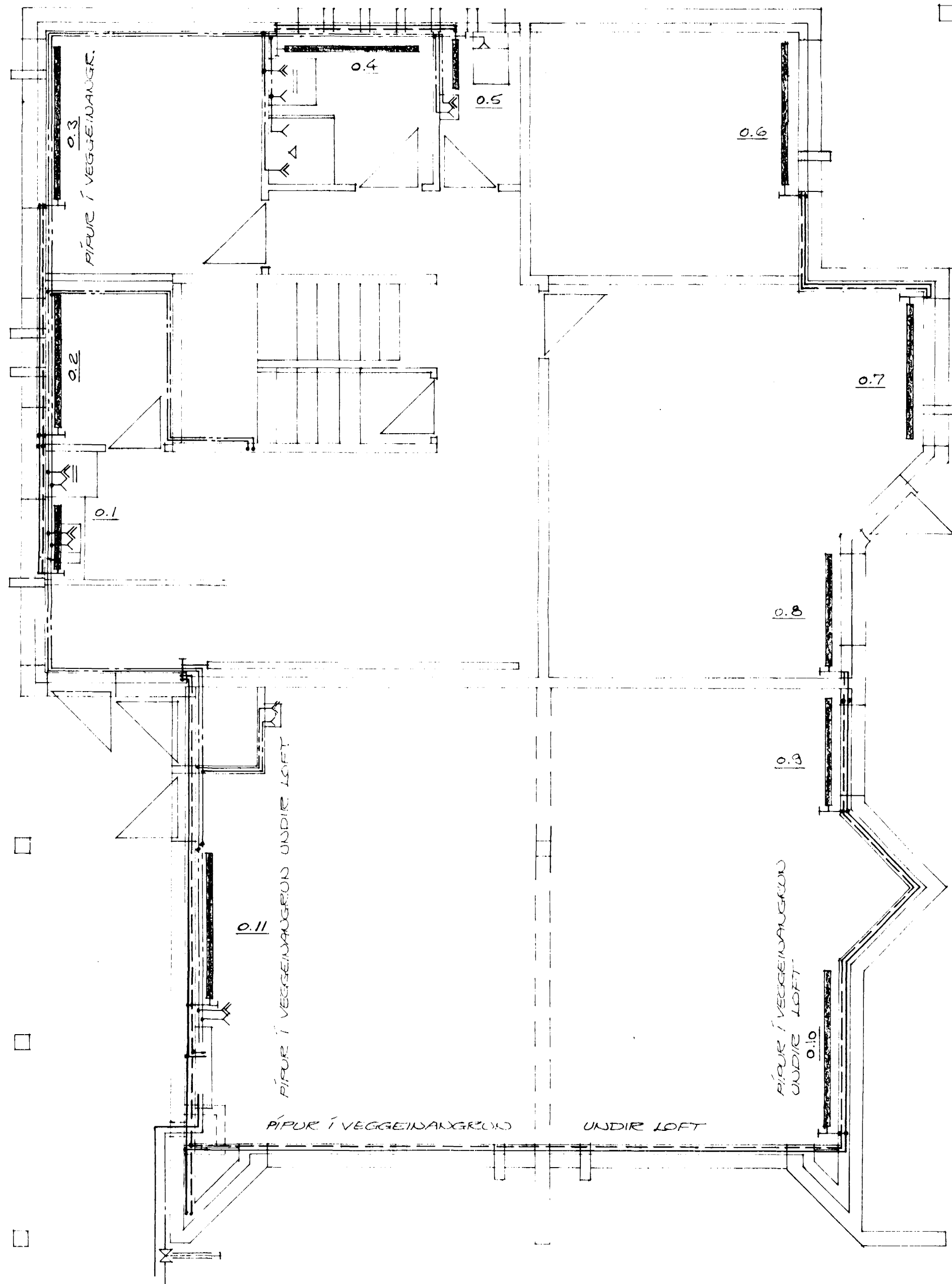
GRUNDMYND KJALLARA, M=1:50
