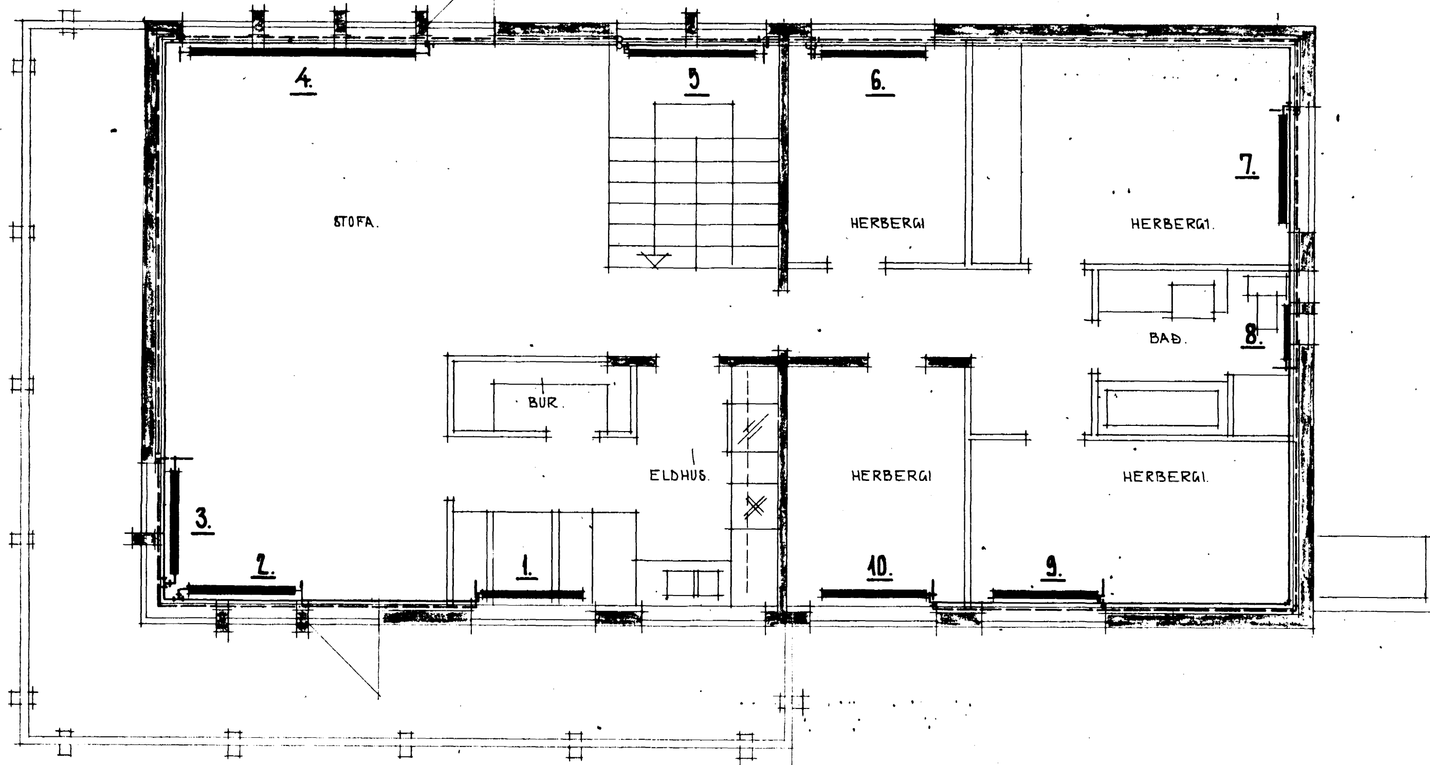
GRUNNMYND EFRI HEDAR_ 1:50_
