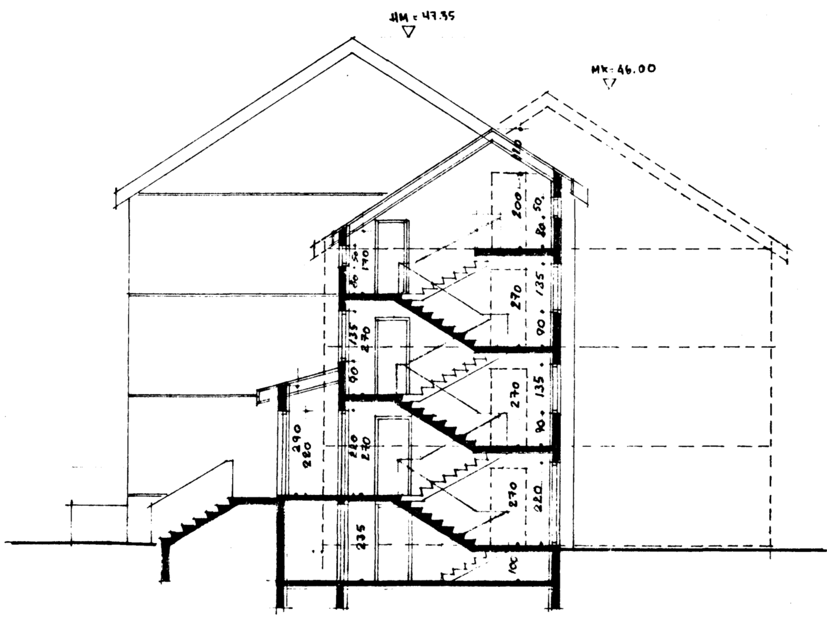
SNÍÐ B-B M. 1:100
