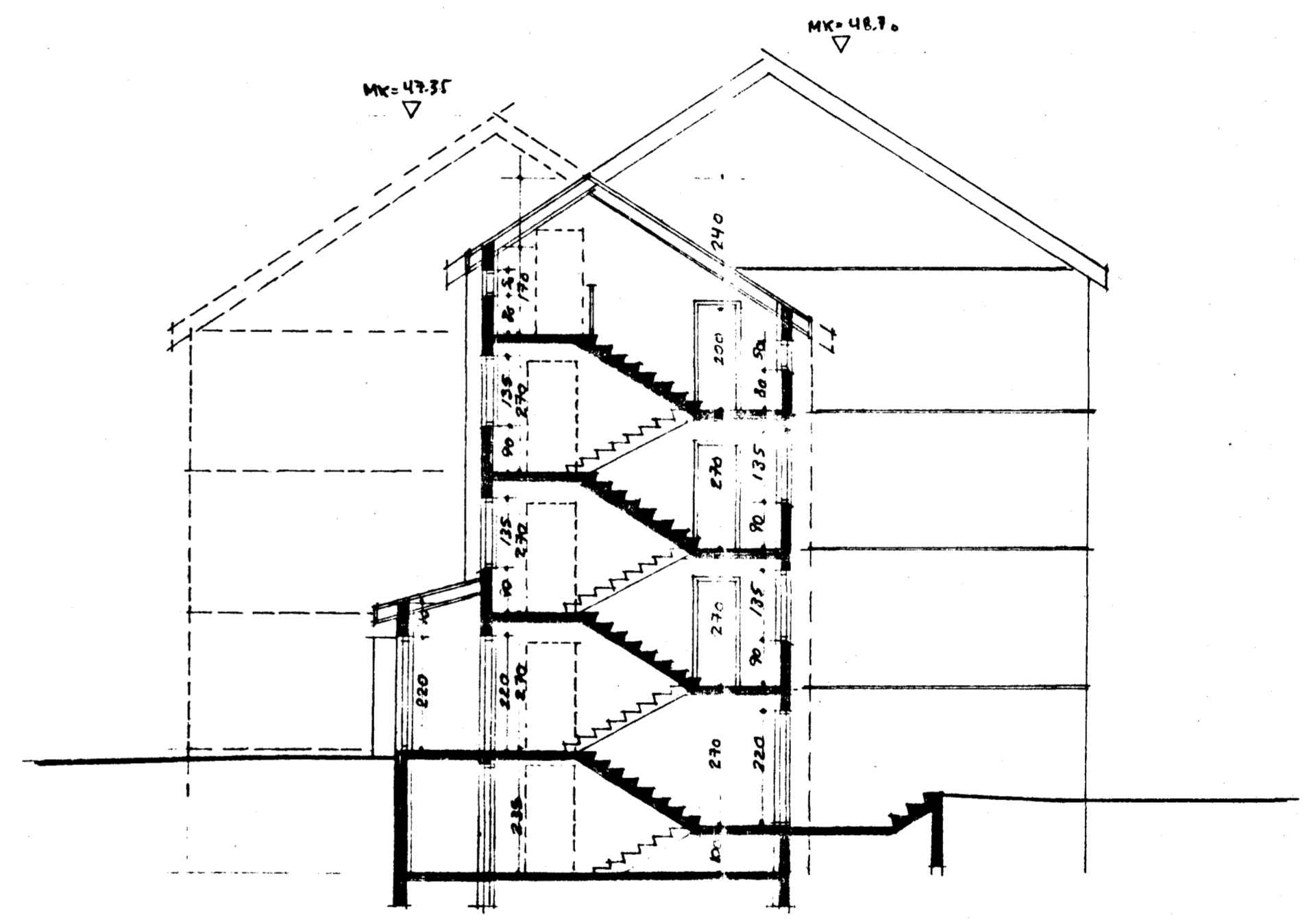
SNÍÐ C-C M. 1:100
