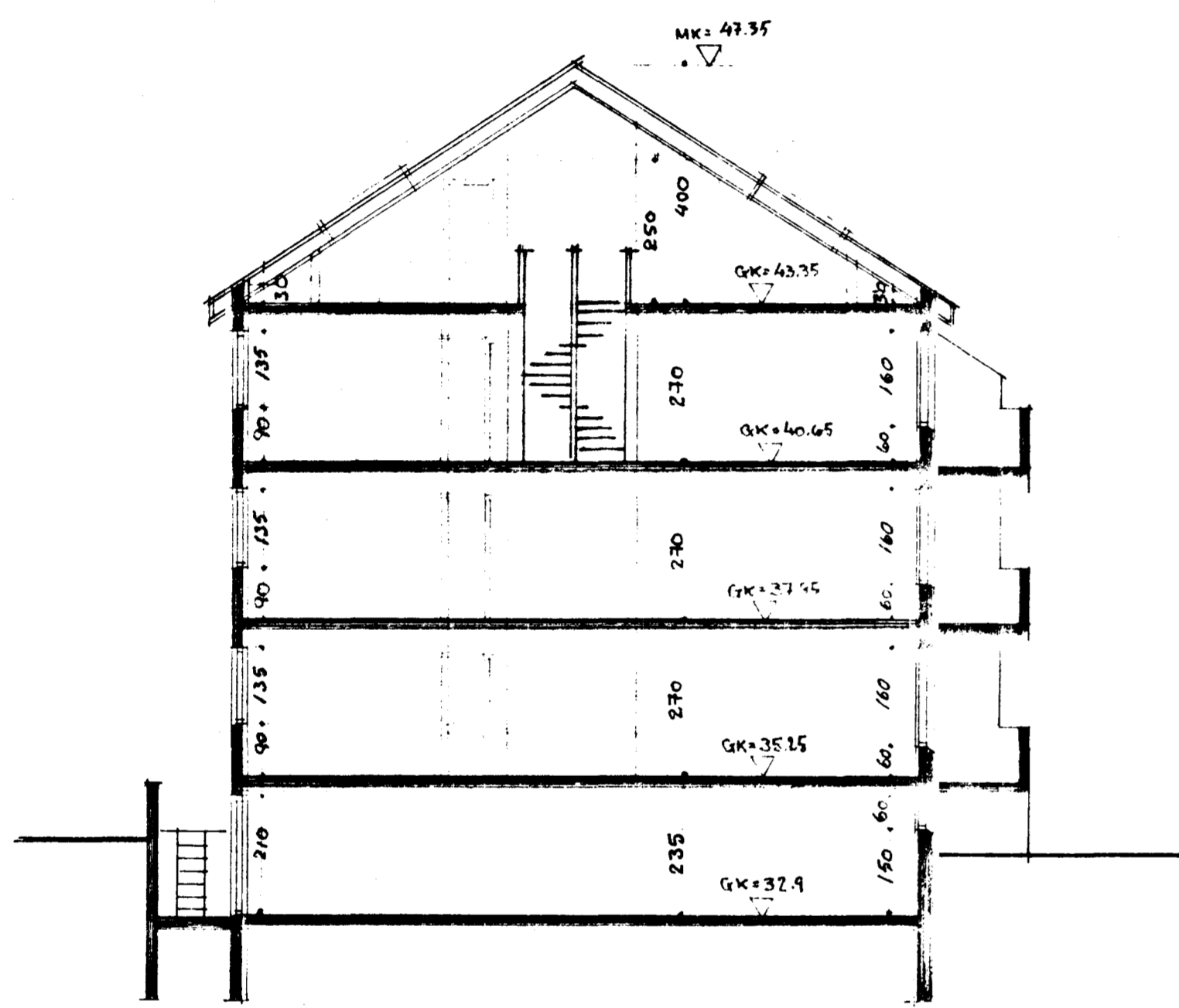
SNÍÐ A-A M. 1:100
