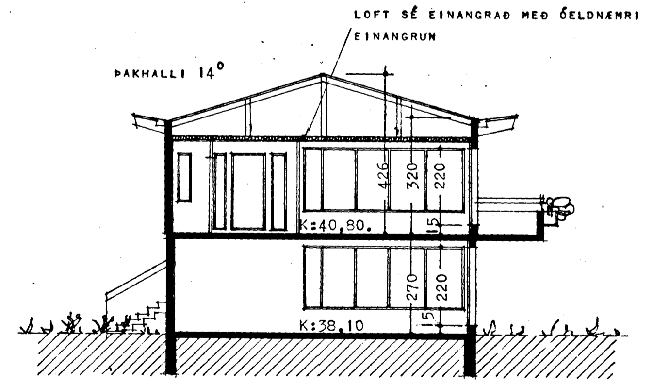
SKURÐUR B - B
