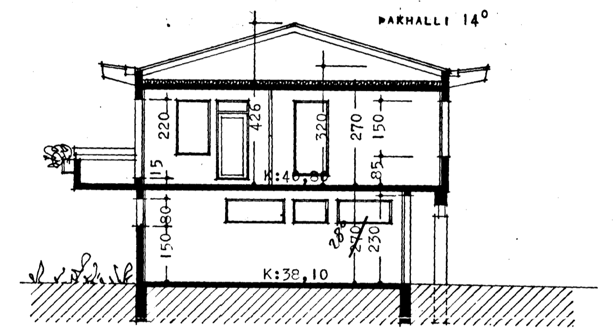
SKURÐUR A - A
