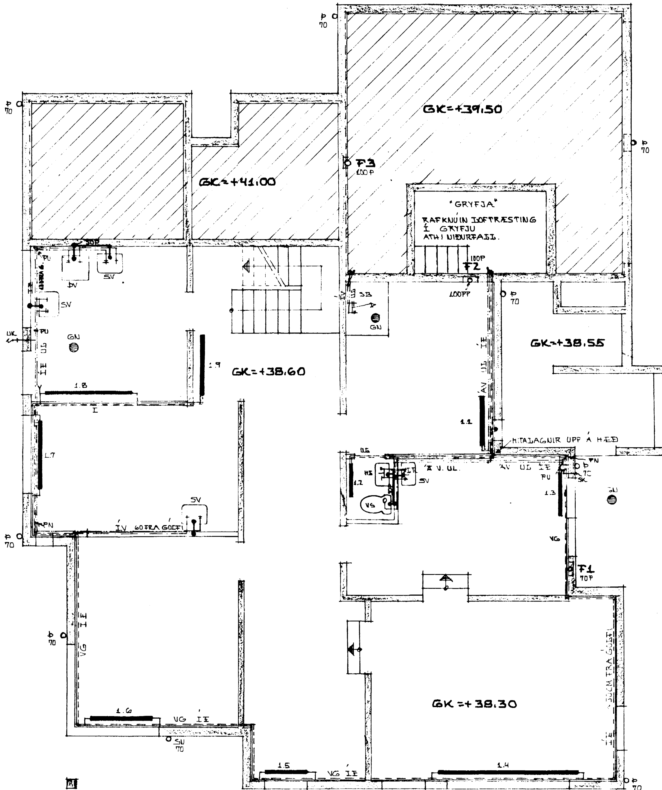
GRUNNMYND 1:50
