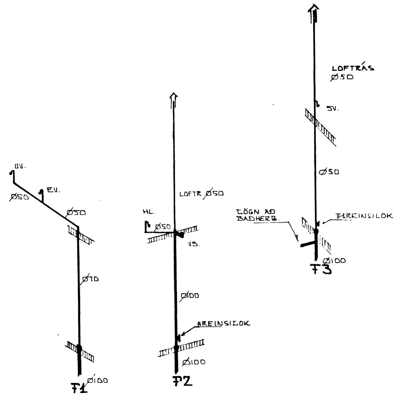
TEKJUFISMYNDIR FRÆKENNLSISSTOFNA 1:50
