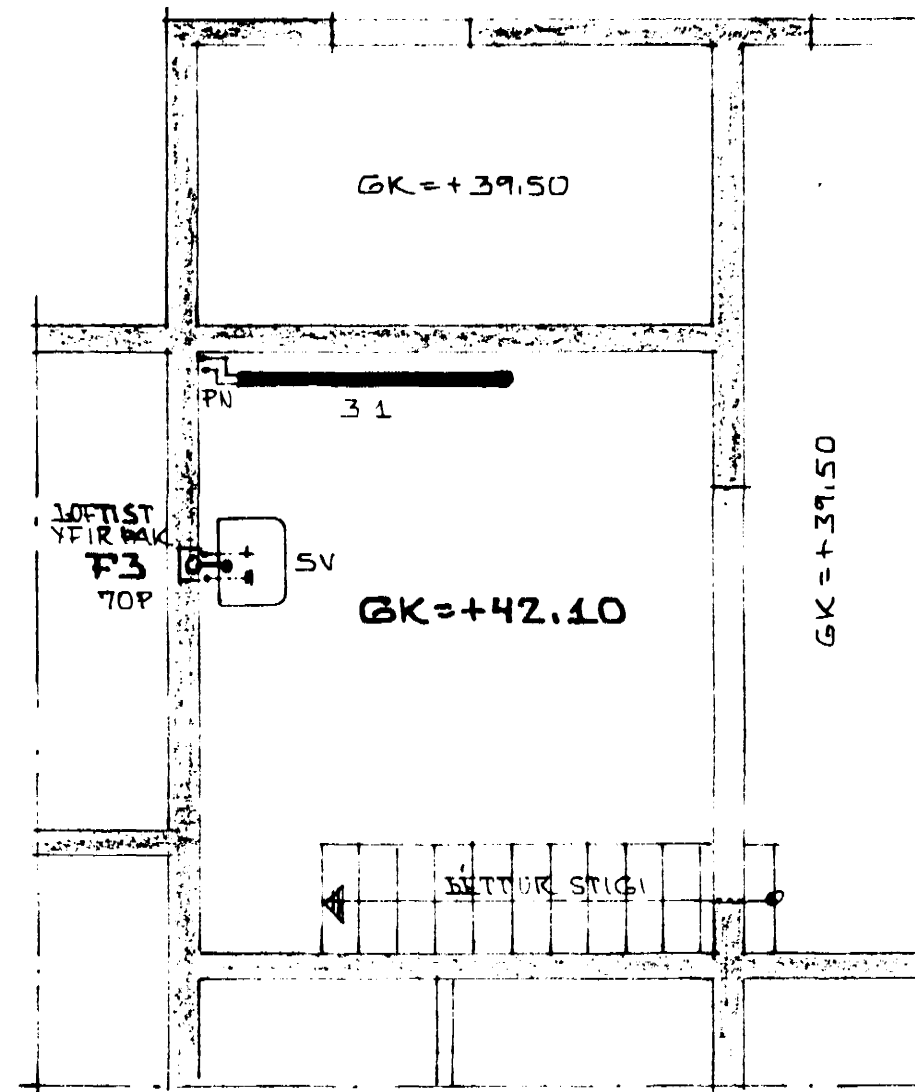
GRUNNMYND RYMIS YFIR BÍLSKUR 1:50
