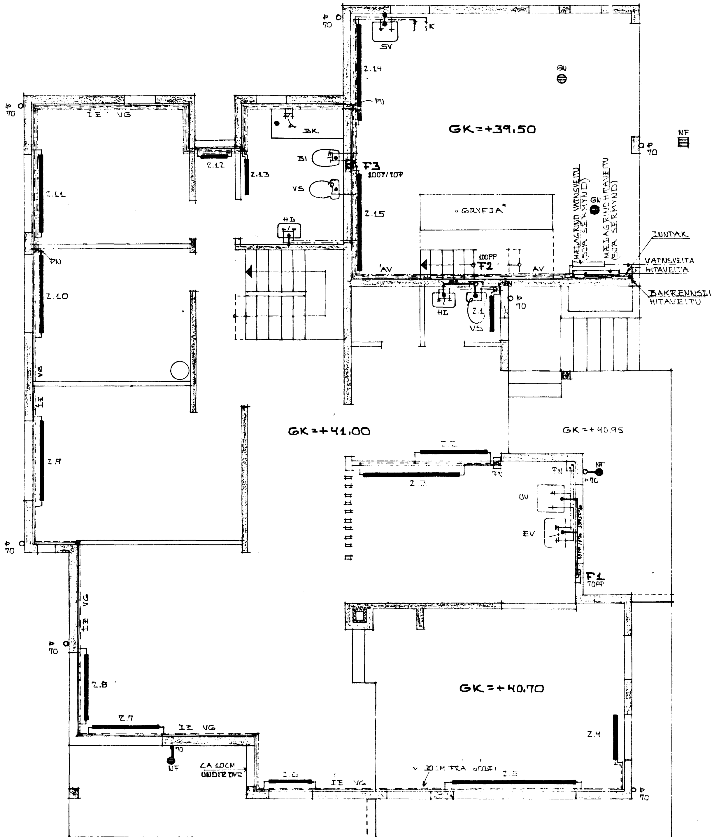
GRUNNMYND 1:50
