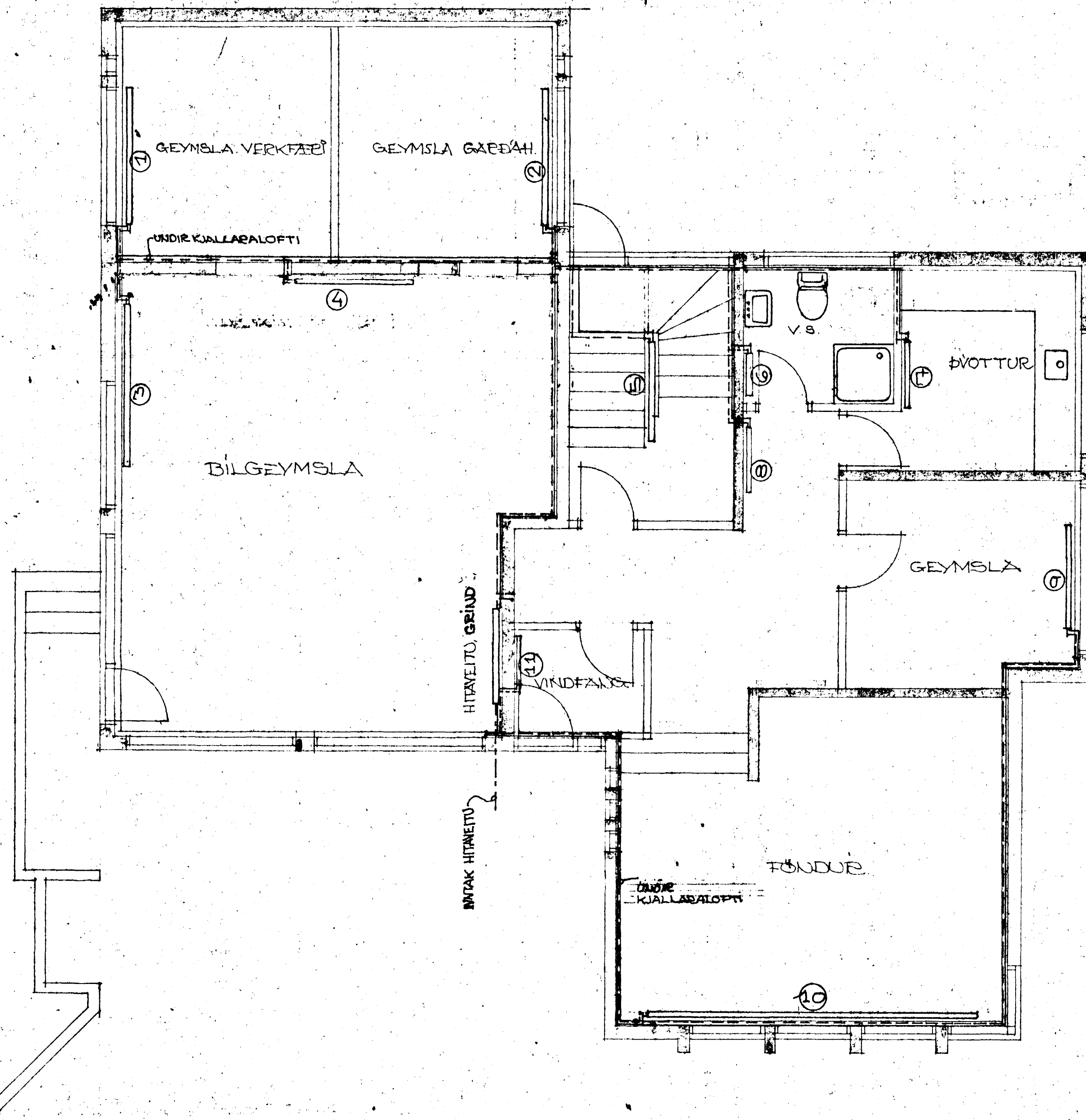
GRUNNMYND KJALLARA M. 1:50.
