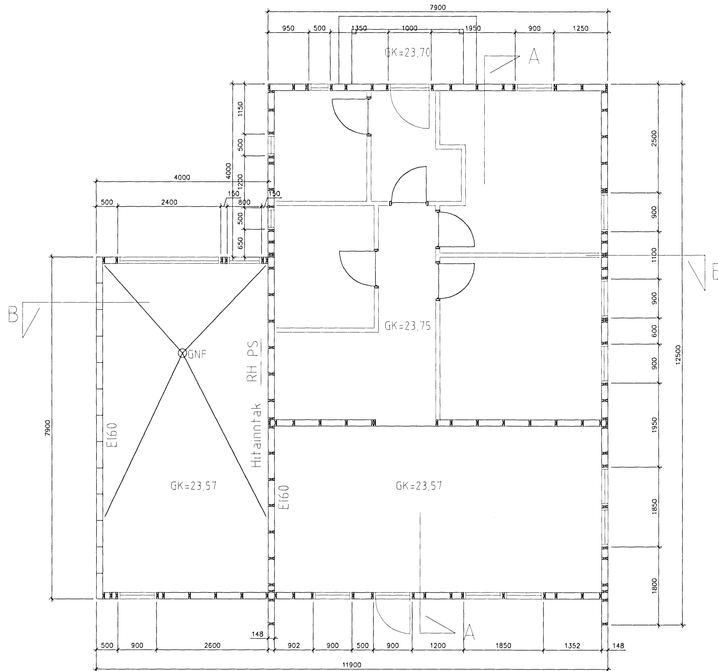
1. HÆÐ Burðargrind Mkv. 1:50
