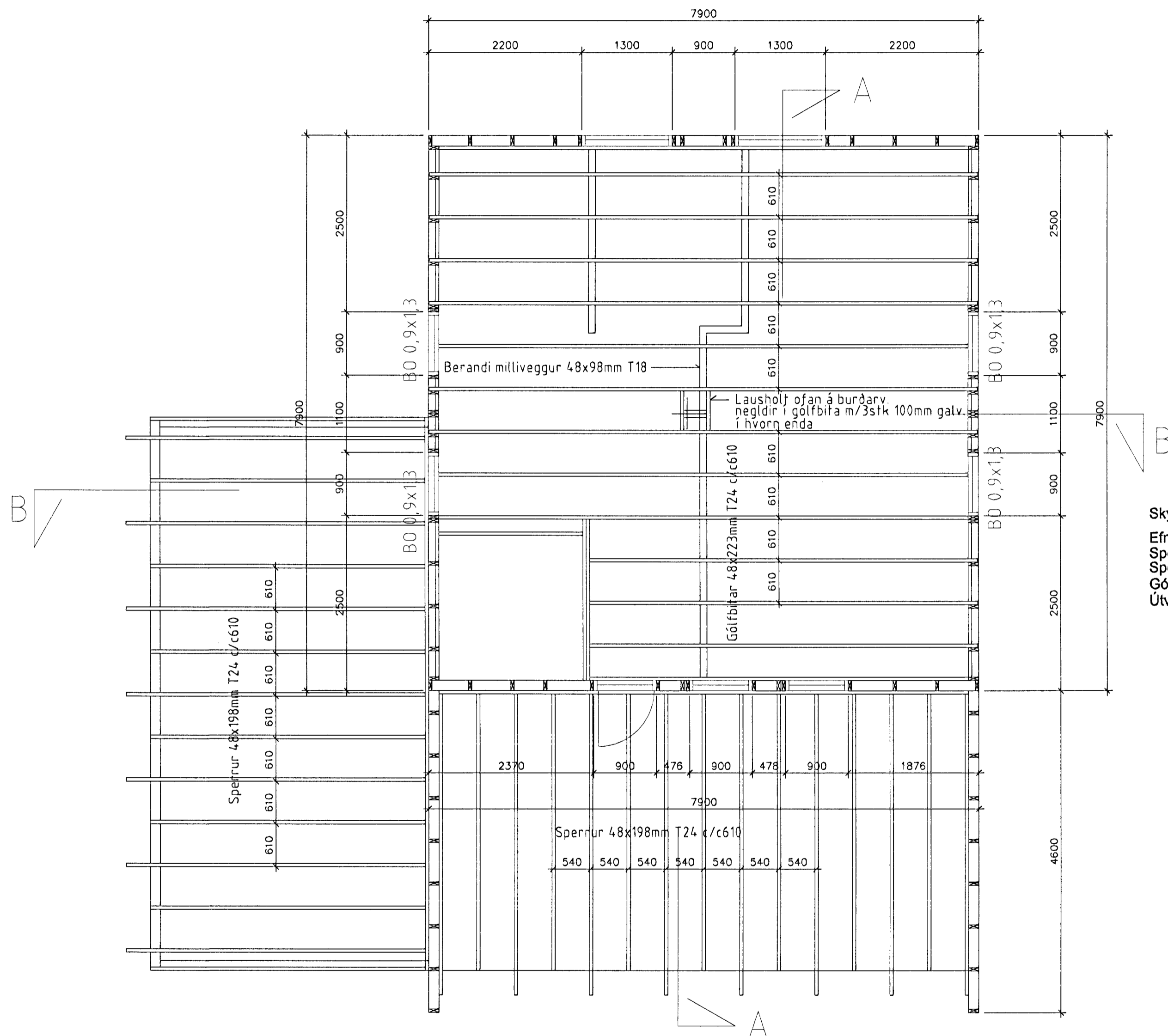
2. HÆÐ Gólfbitar og sperrur á lágbyggingu Mkv. 1:50
