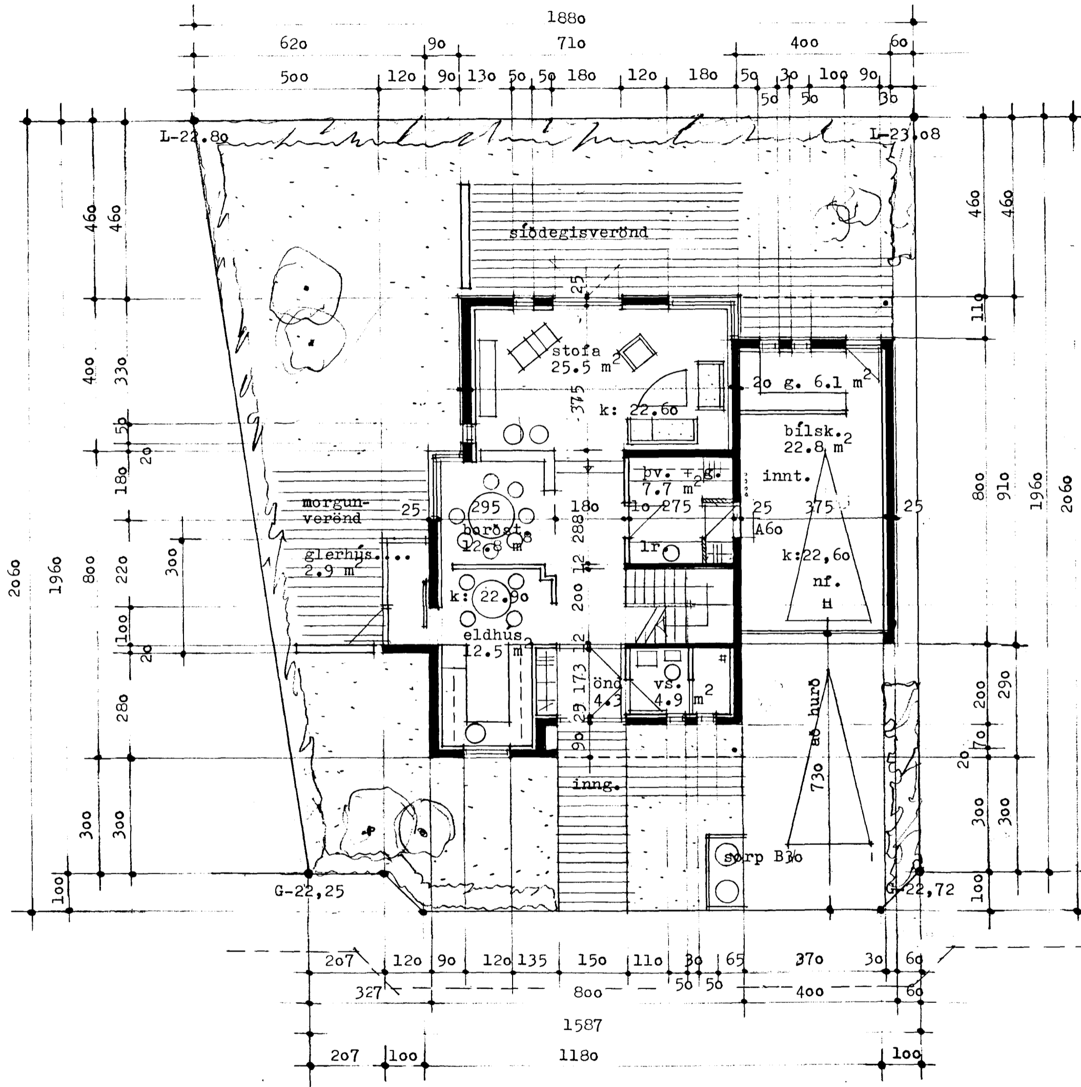
grunnmynd 1.hæð 1:100
