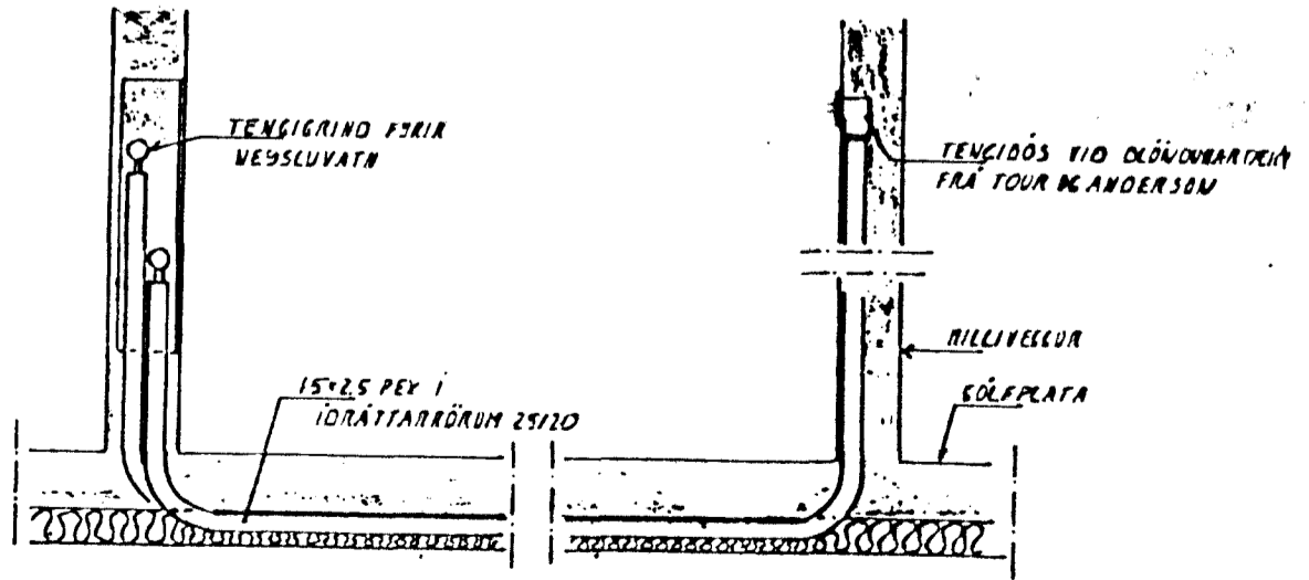
TENGING NEYSLUVATNSLAGNA
