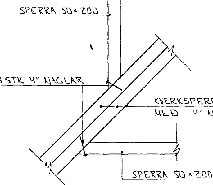
SÉRMYND A · 1:10
