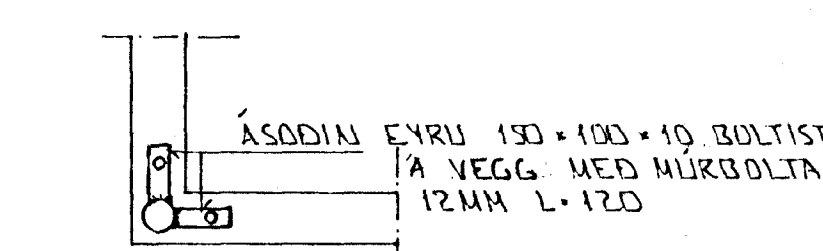
SNID X-X · 1:20
