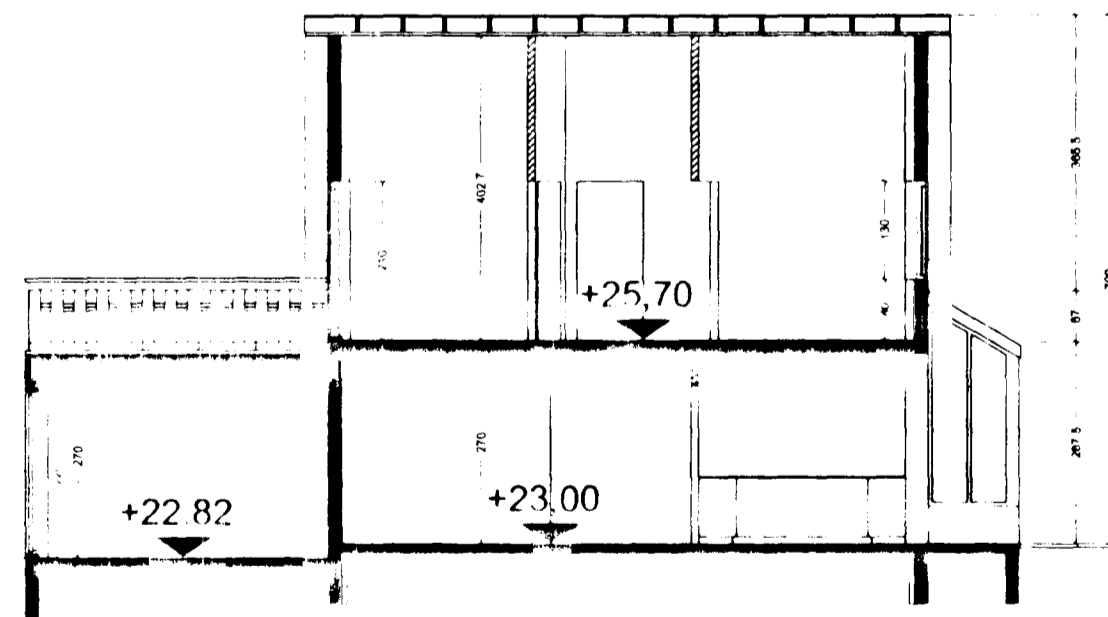
SKURÐUR A-A
