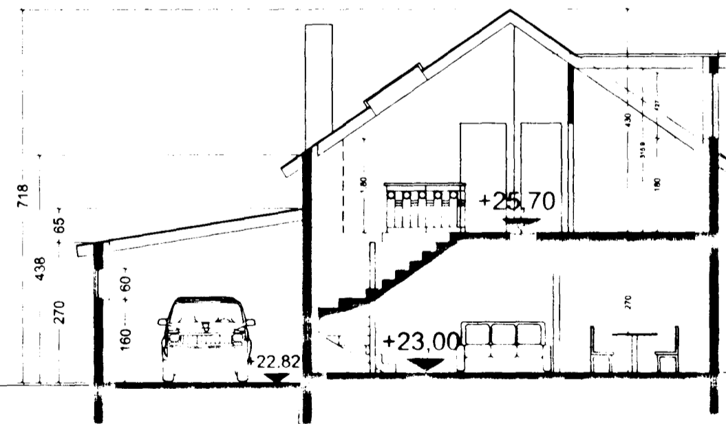
SKURÐUR B-B
