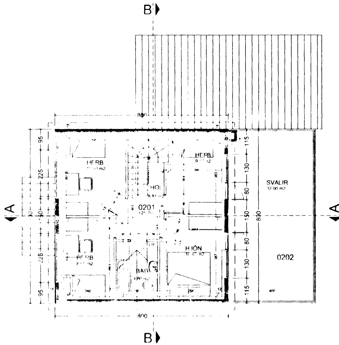
GRUNNMYND EFRI HÆÐ
