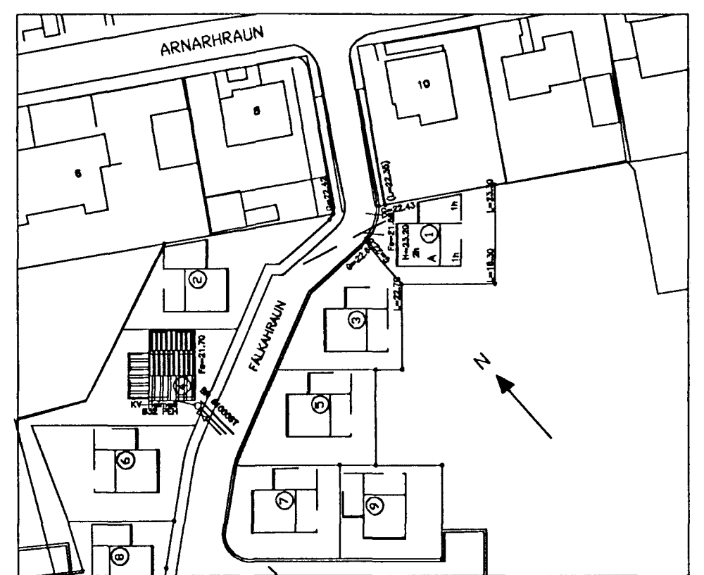
Afstöðumynd mkv.1:500
