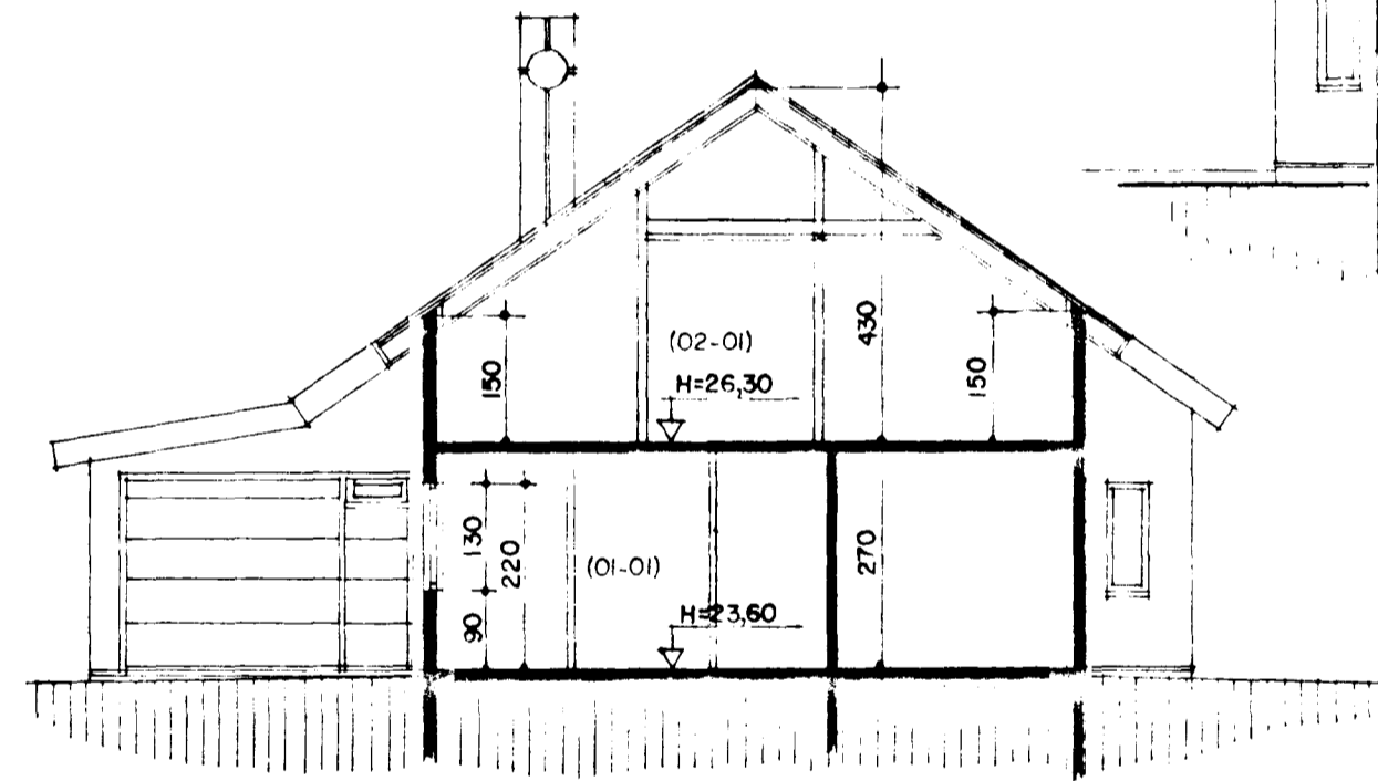
SNEIÐING B-B MKV. 1:100.
