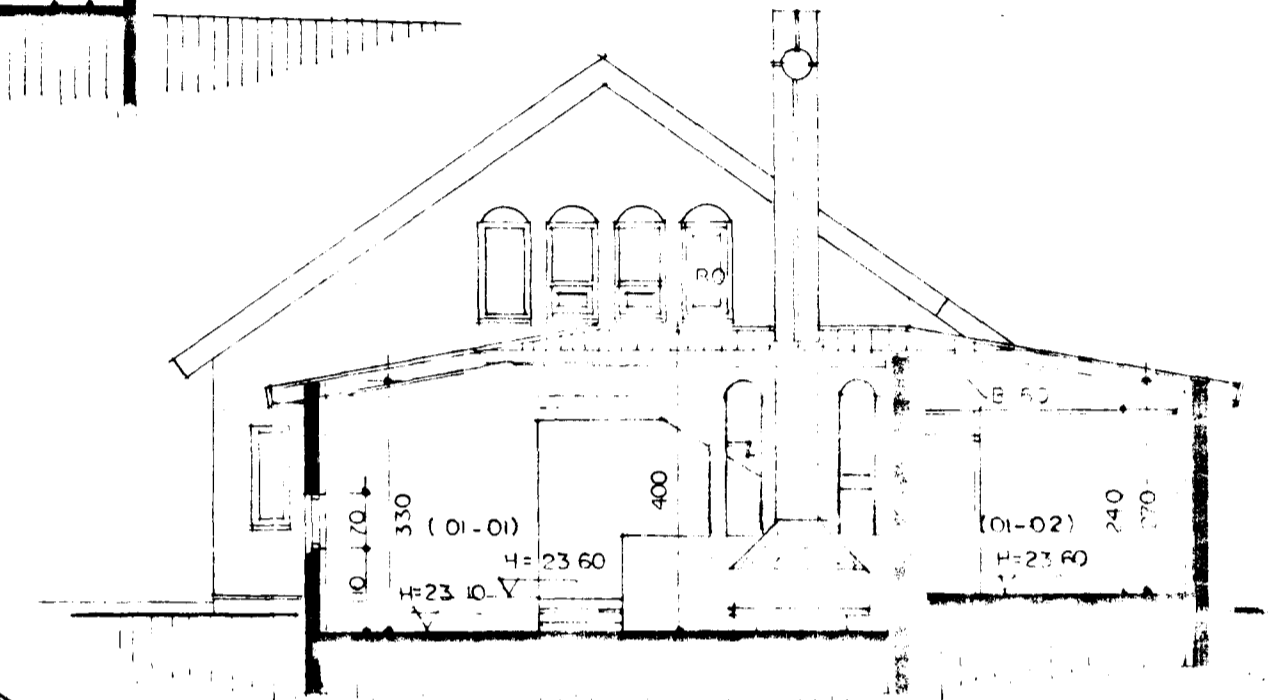
SNEIÐING C-C MKV. 1:100.
