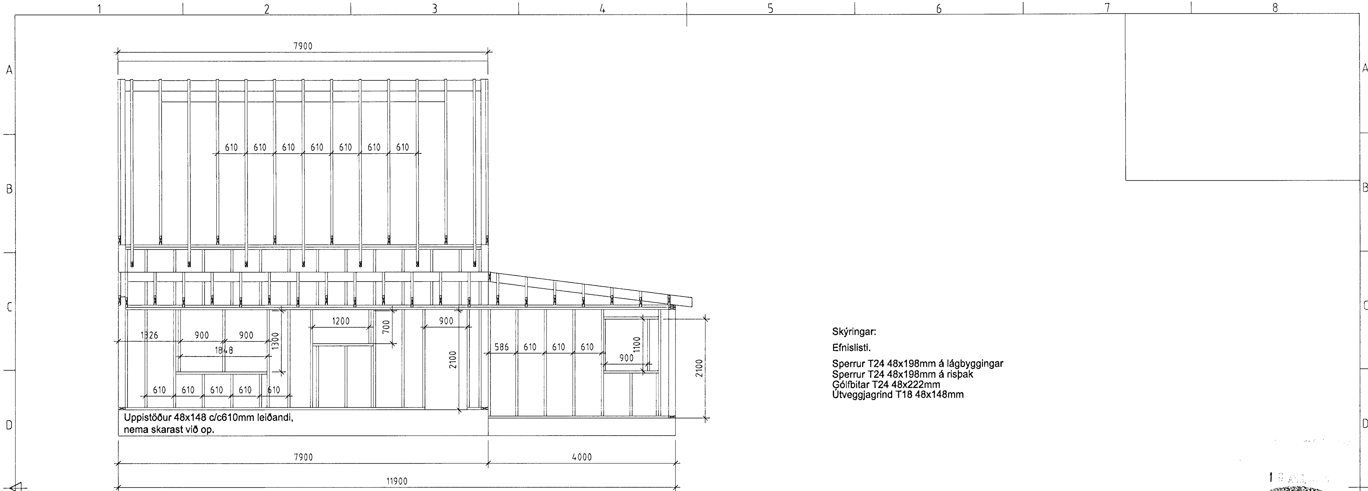
NORÐUR Mkv. 1:50
