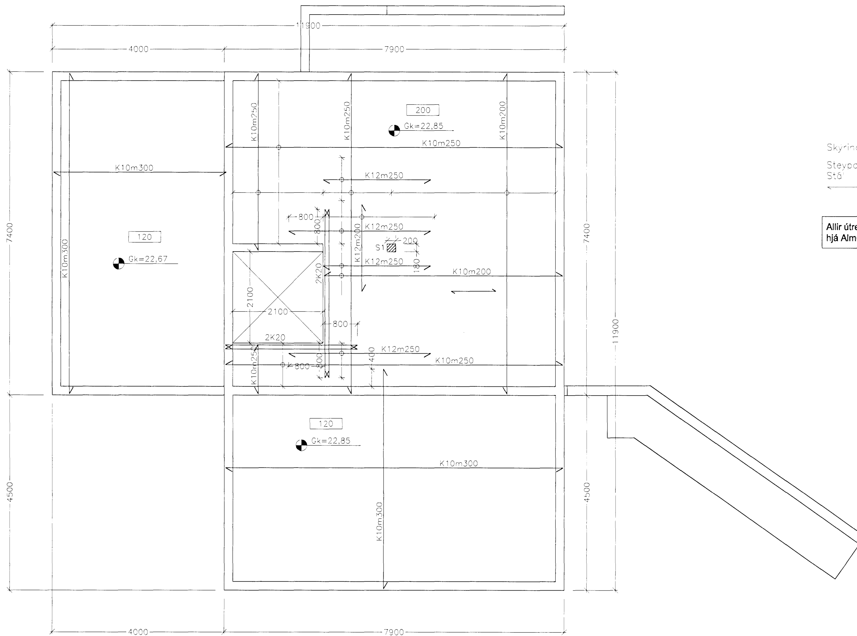
Steypt plata 1.Hæð Mkv. 1:50
