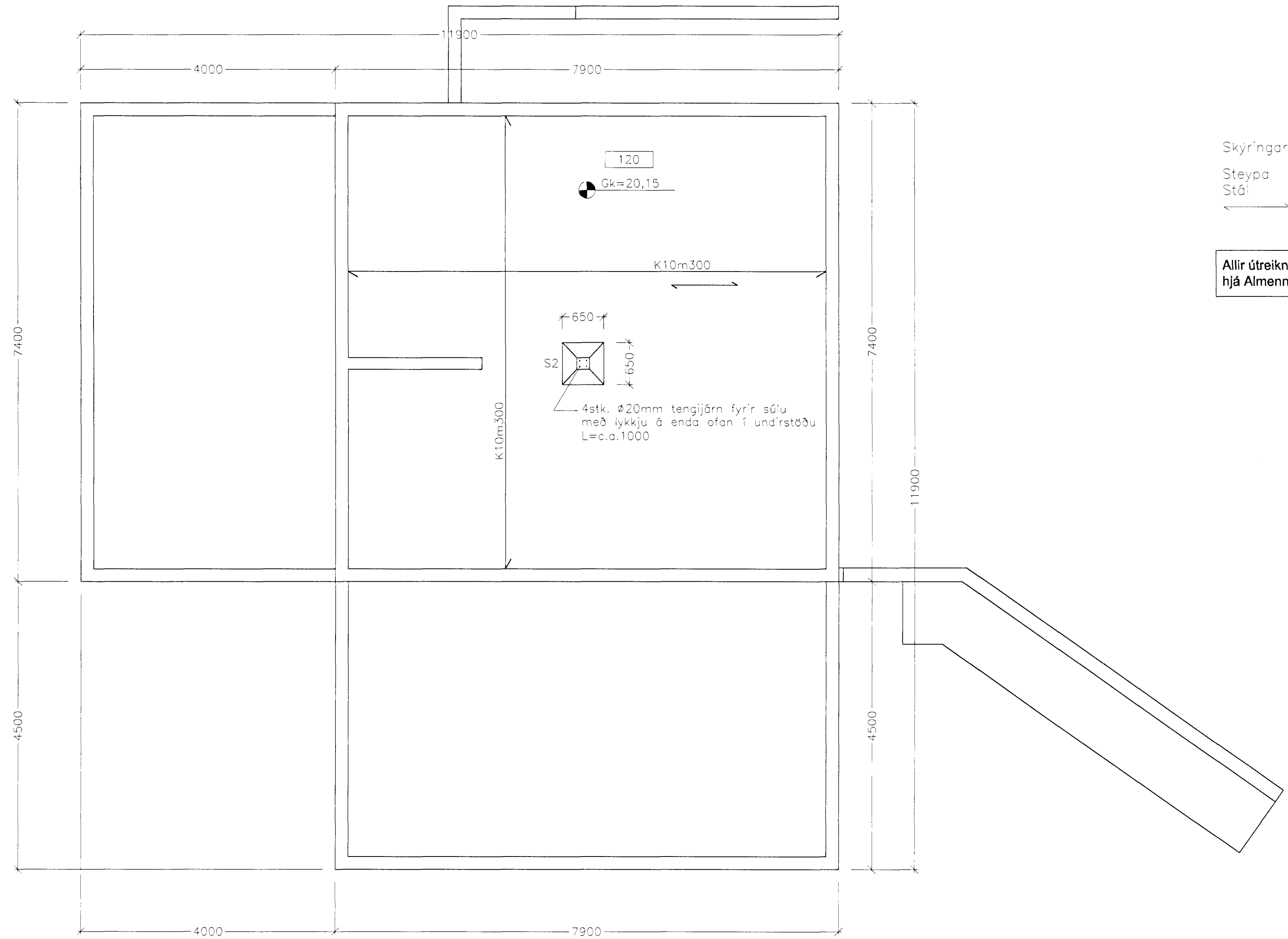
Botnplata, Jarðhæð Mkv. 1:50
