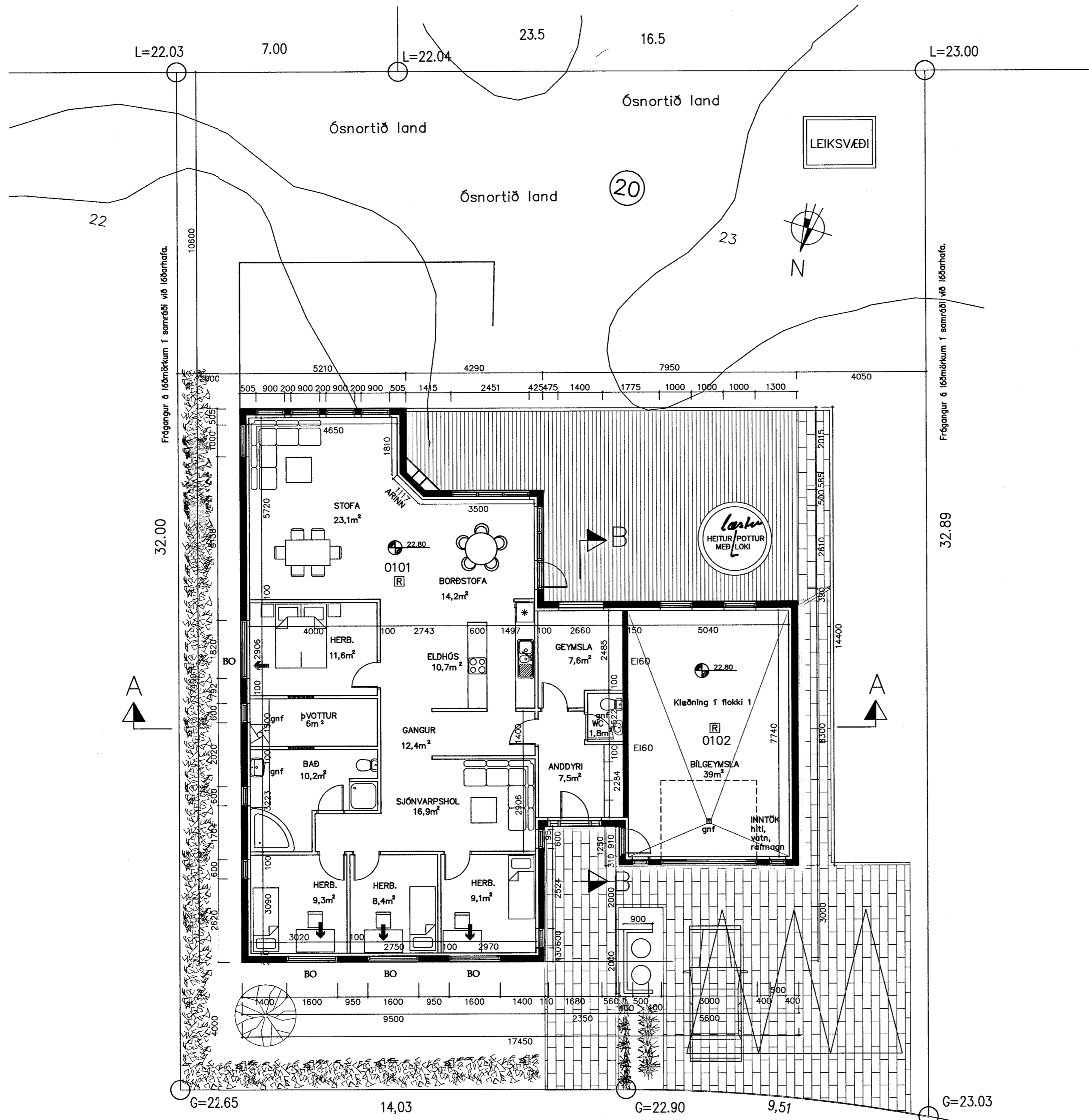
GRUNNMYND 1:100
