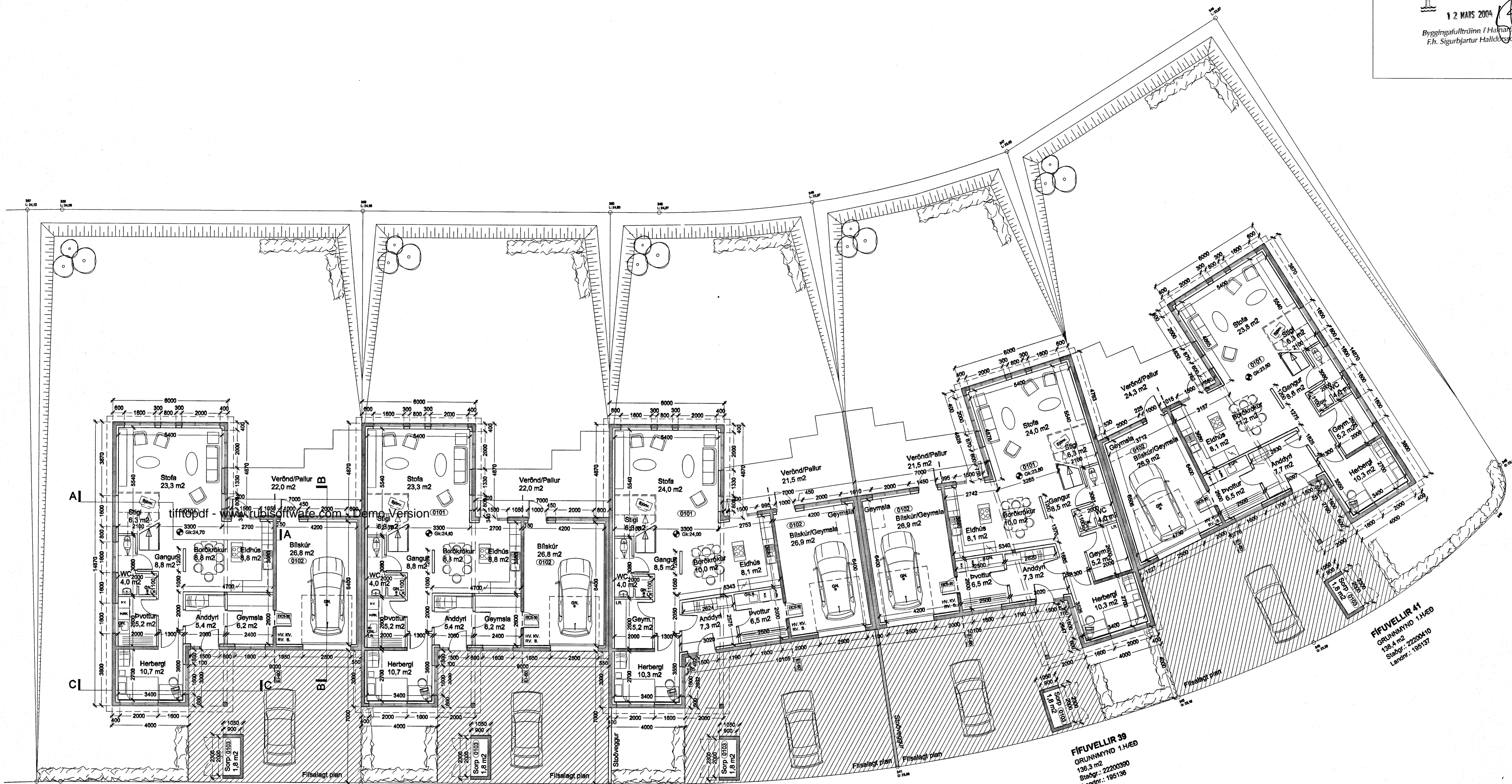
FÍFUVELLIR 33 GRUNNMÝND 1.HÆÐ 132,2 m 2 Staðgr.: 22200330 Landnr.: 195132
