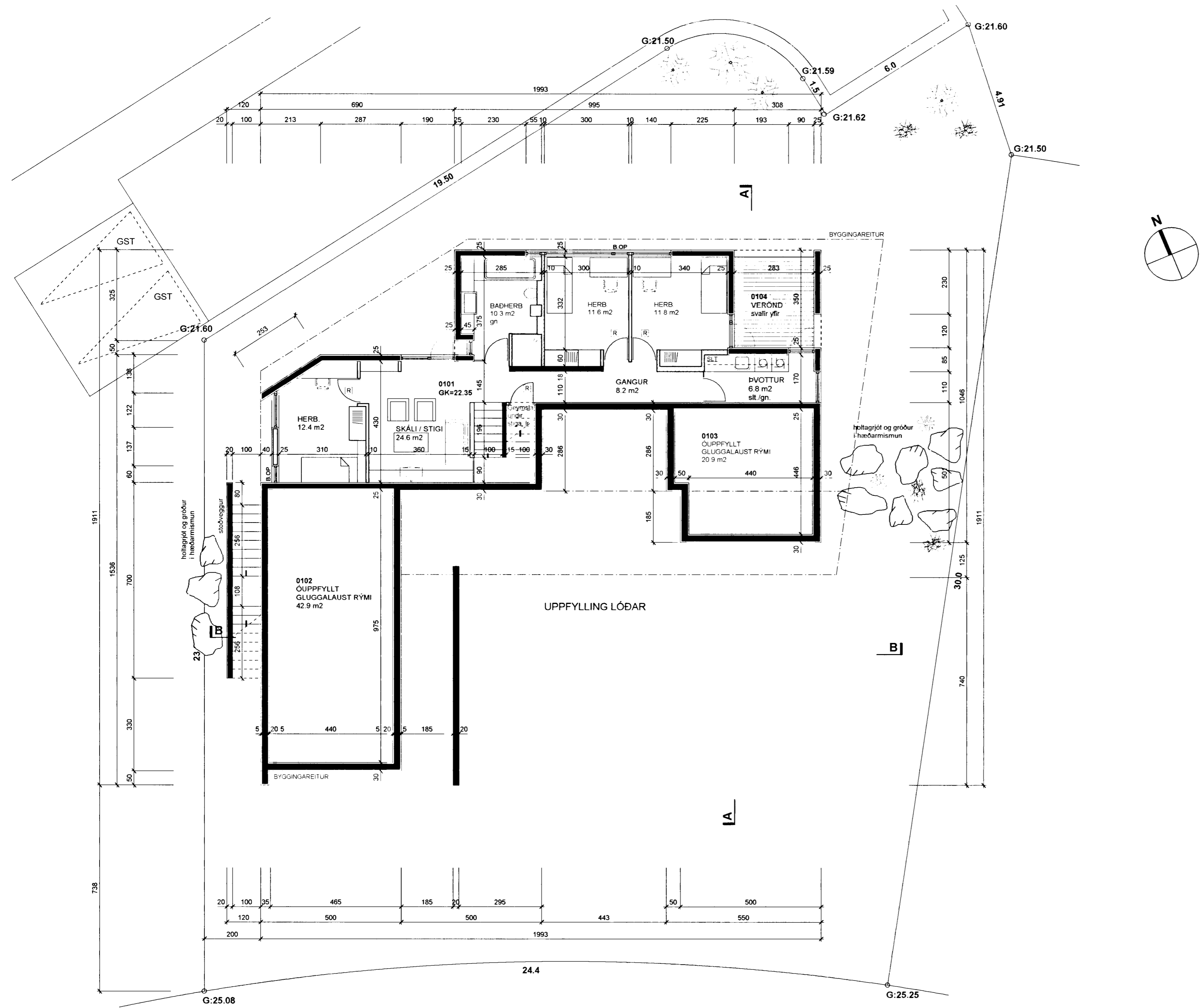
GRUNNMYND NEÐRI HÆÐAR
