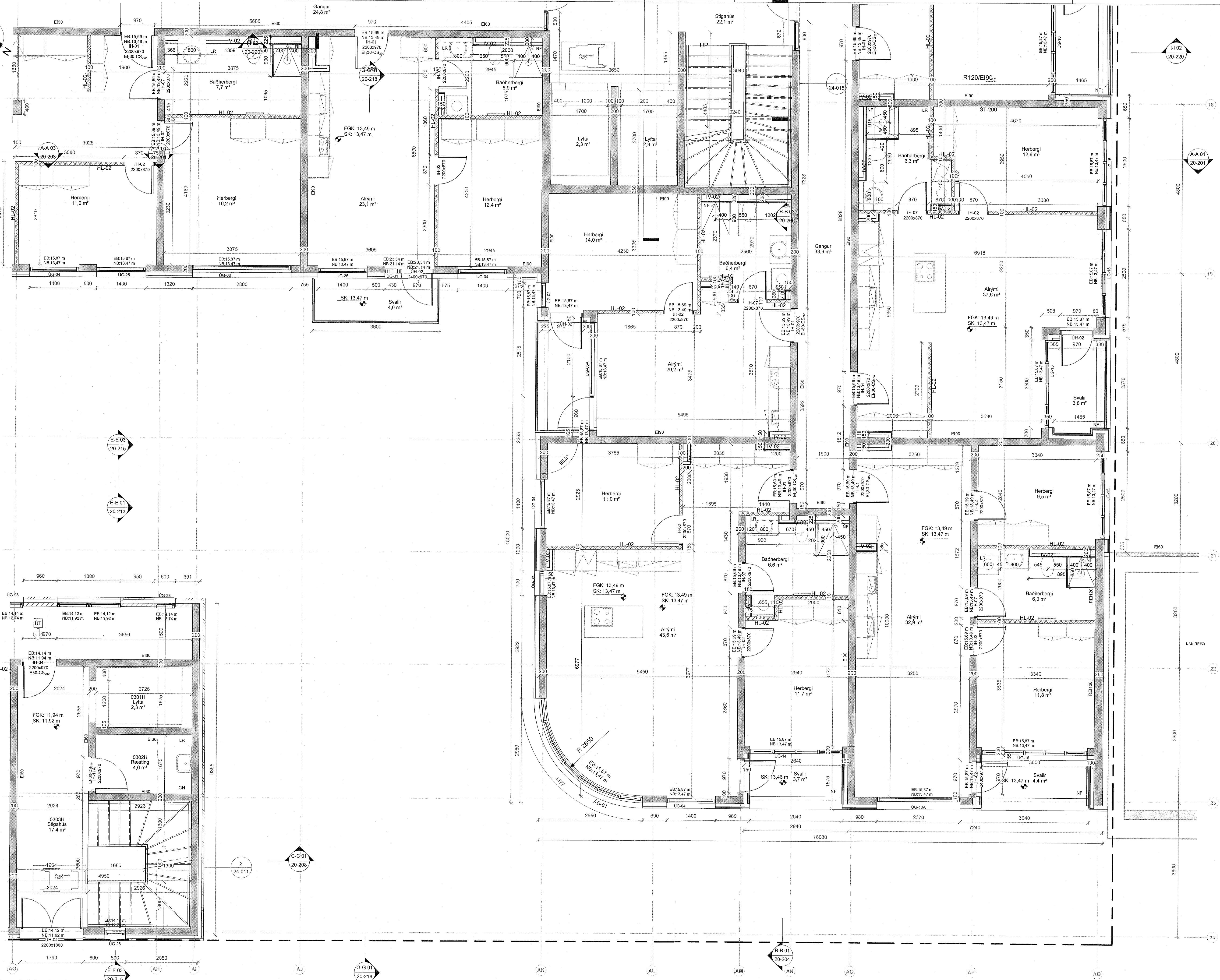
1 3. hæð Verk. 1-50 - 02 1:50
