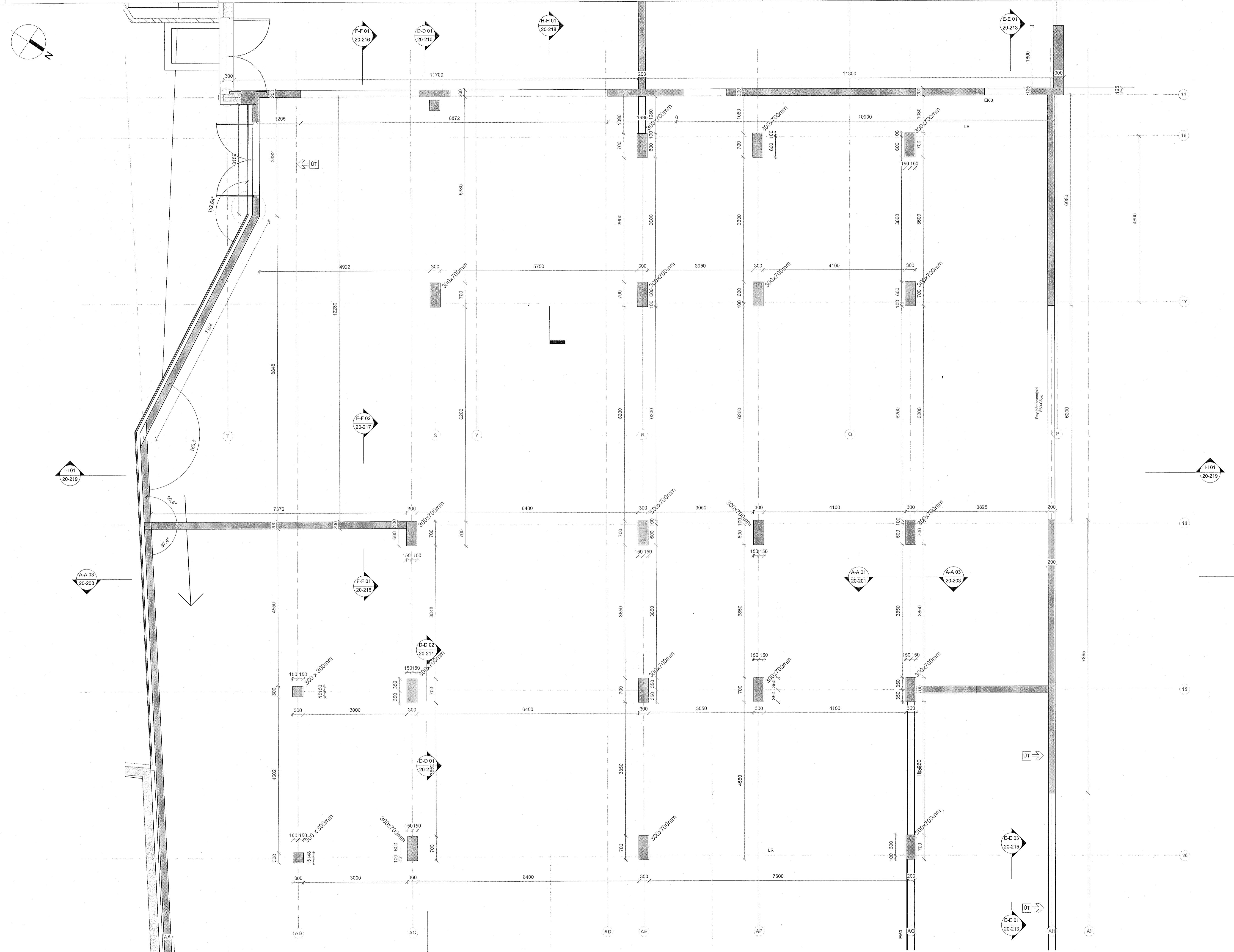
1. hæð Verk. 1-50 - 03 1 : 50
