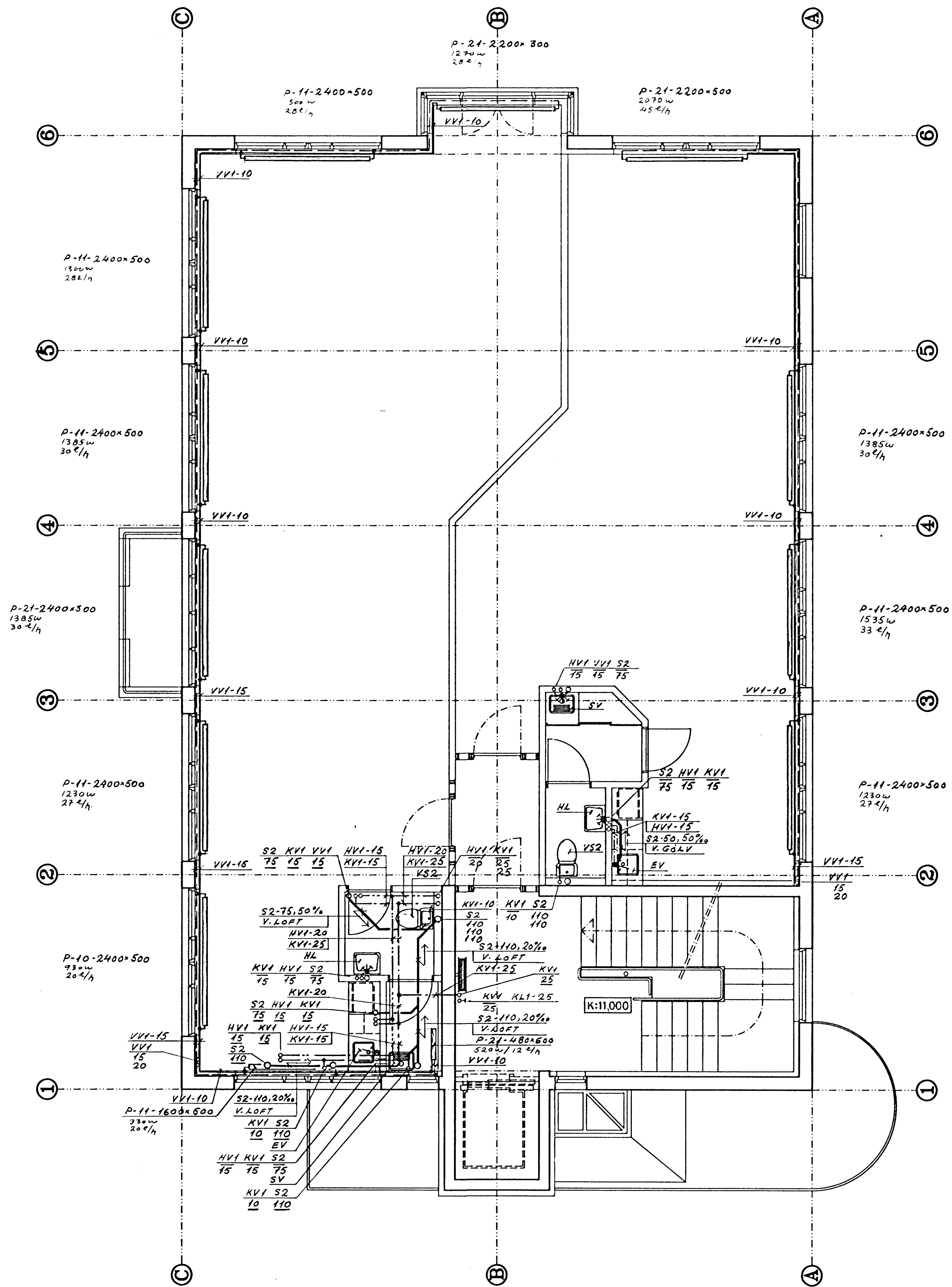
3. HÆÐ
