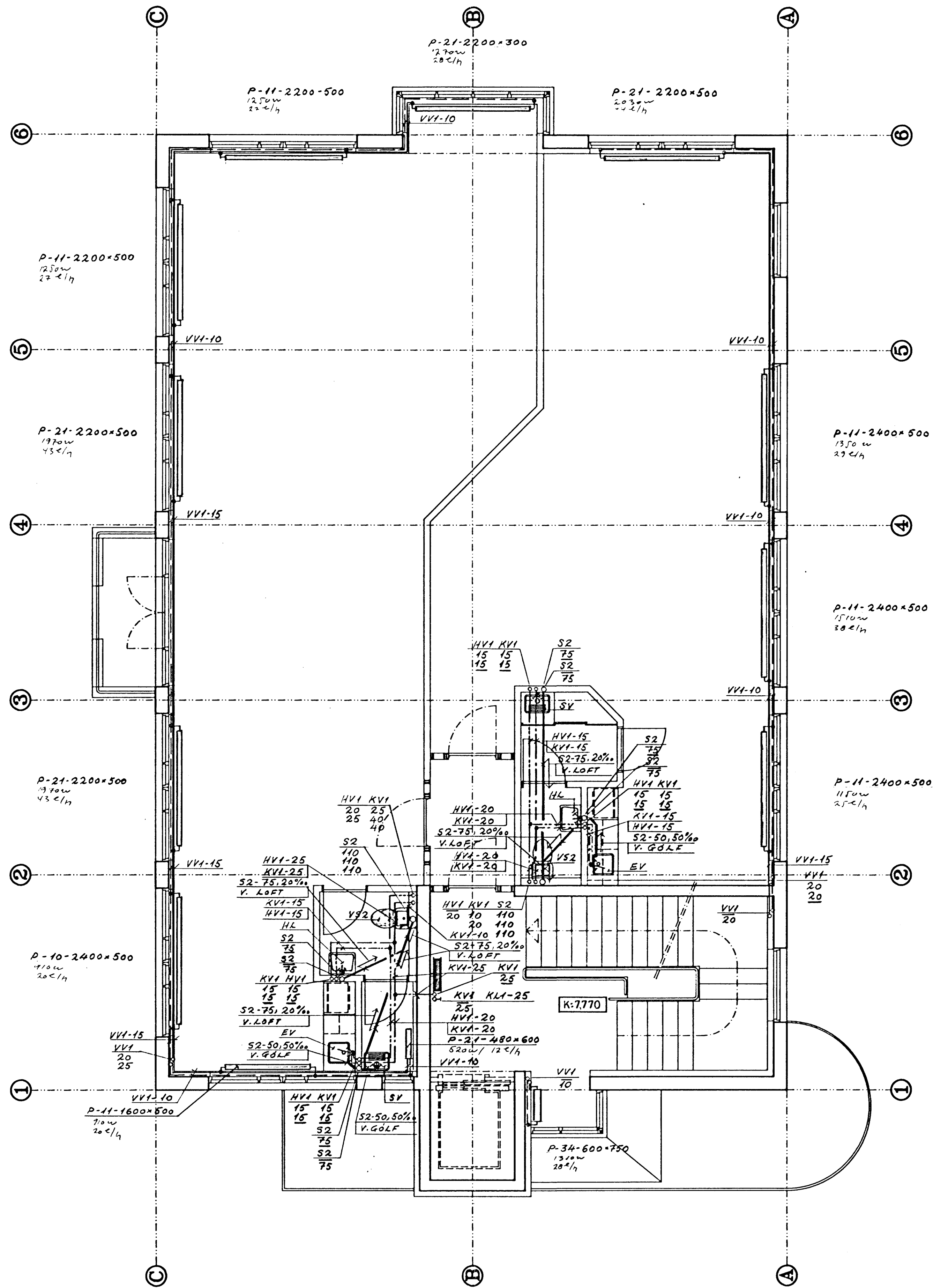
2. HÆÐ
