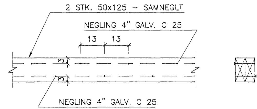
SAMNEGLING TVÖFALDRA STODA 1:10
