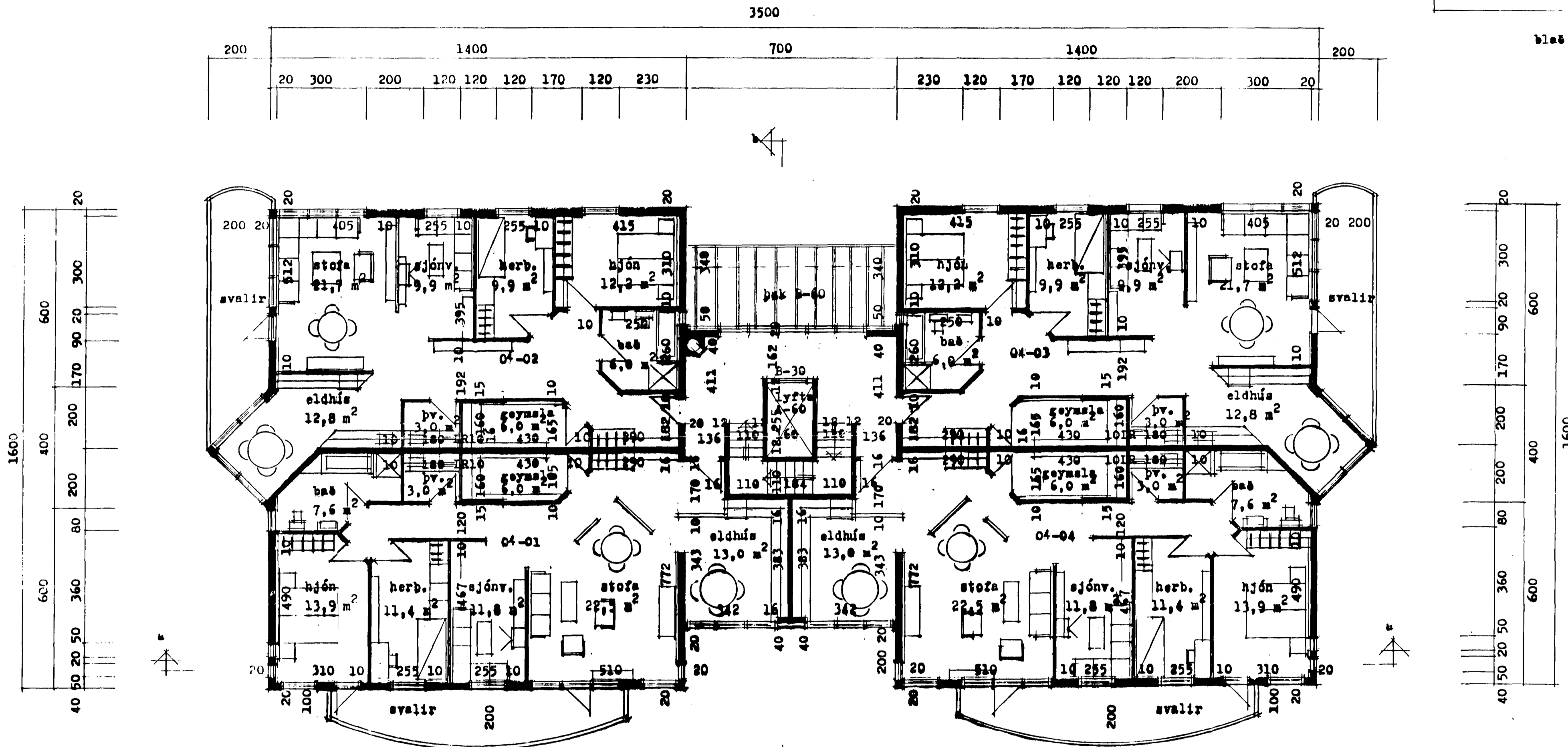
grunnmynd 4. hæðar
