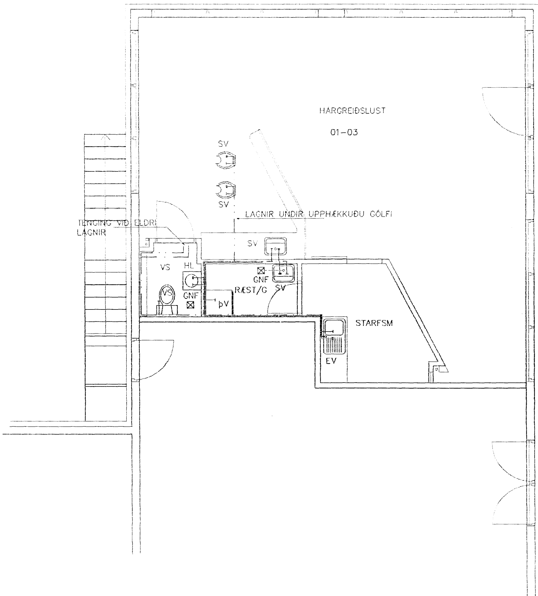
GRUNNMYND 1 HÆÐ 1:50
