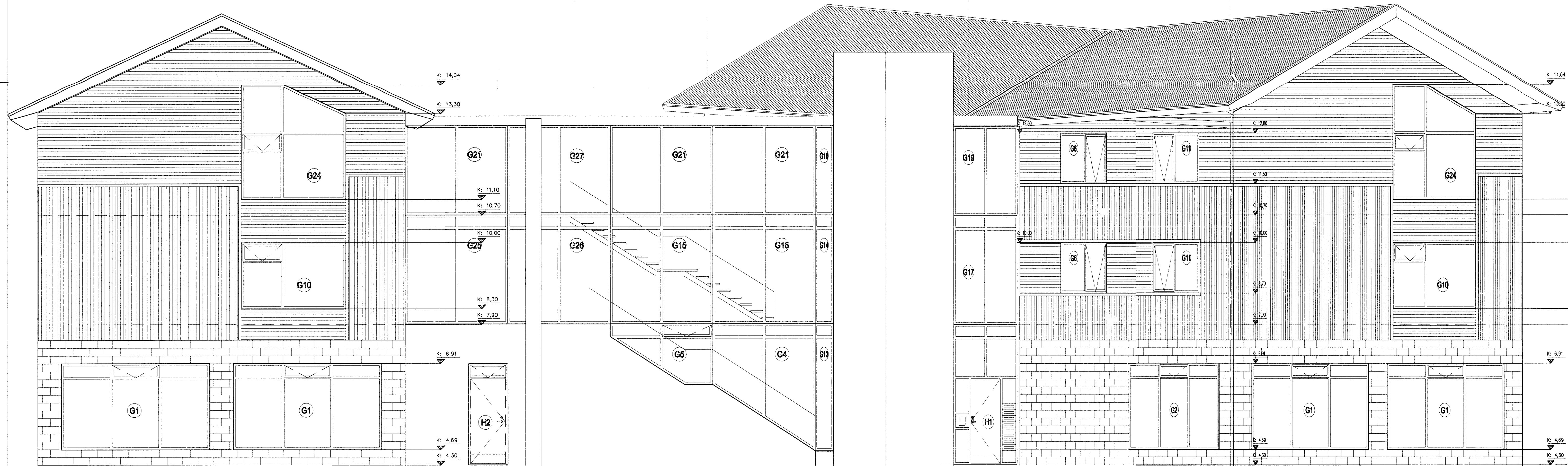
NORÐURHLIÐ
