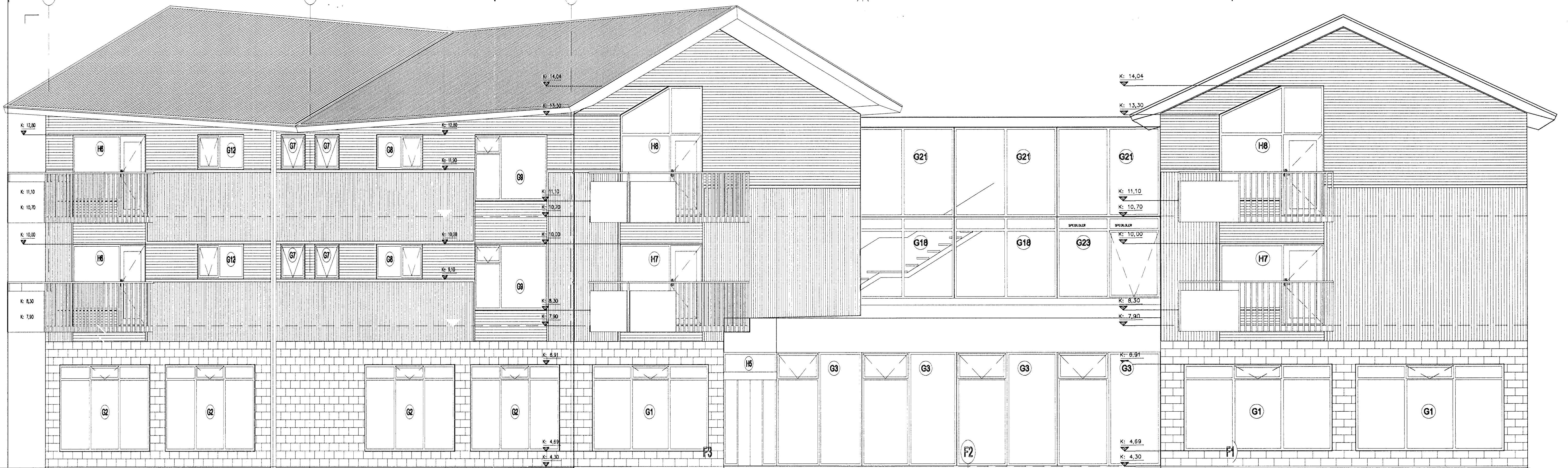
SUÐURHLIÐ
