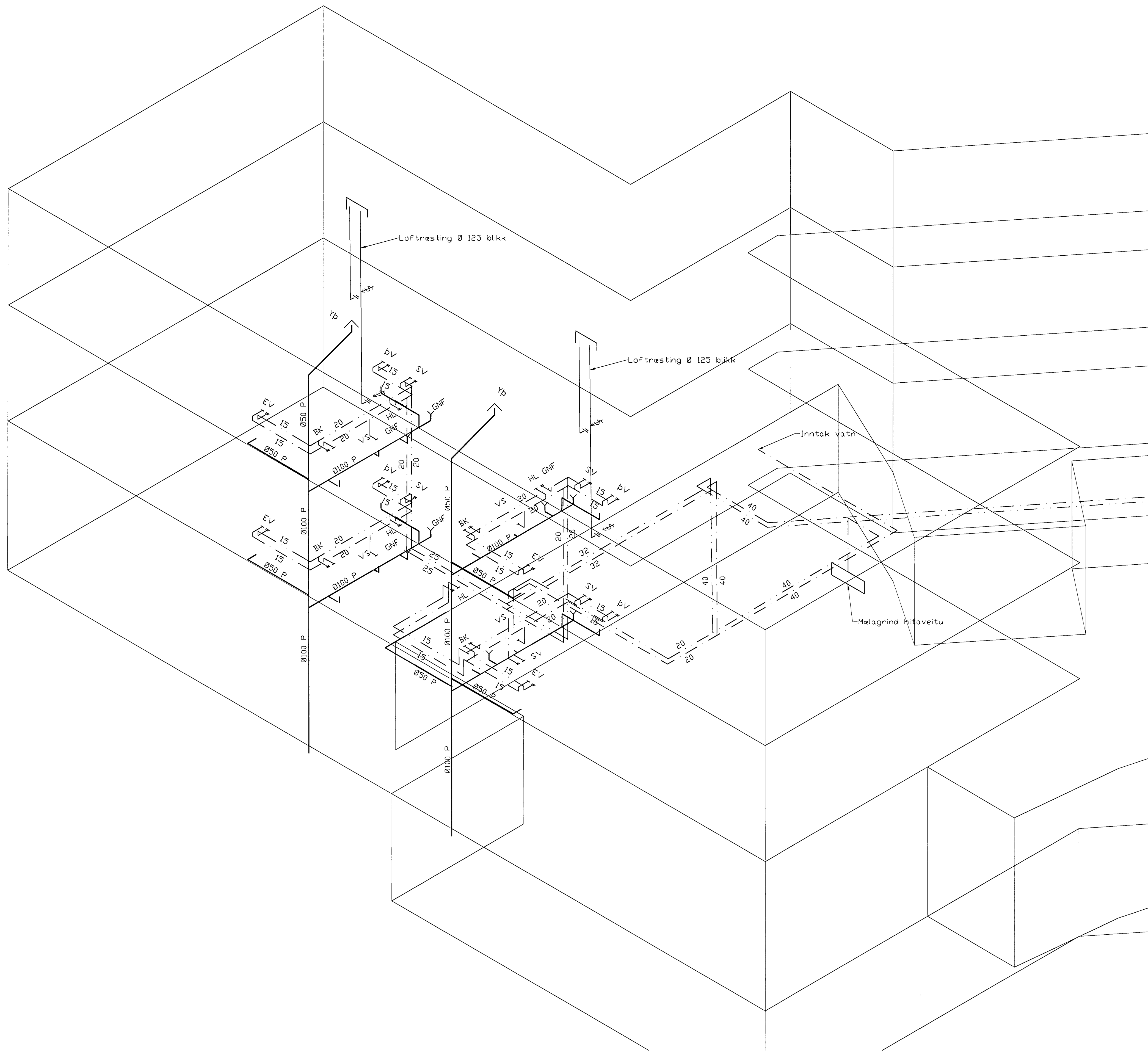
Vatns- og frárennislagnir, Rúmmynd, 1:50
