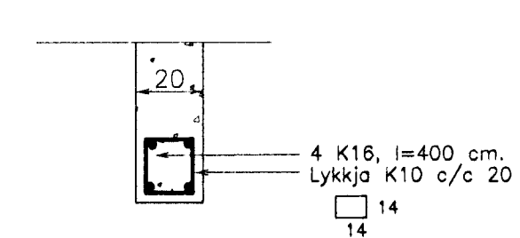
S2.6. Sála S2.6. 1:20. 8 | 9
