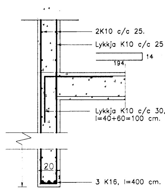
B2.2. Bíti B2.2. 1:20. 8 | 9
