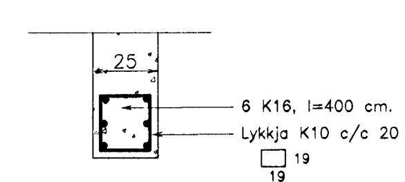
S2.5. Sála S2.5. 1:20. 8 | 9
