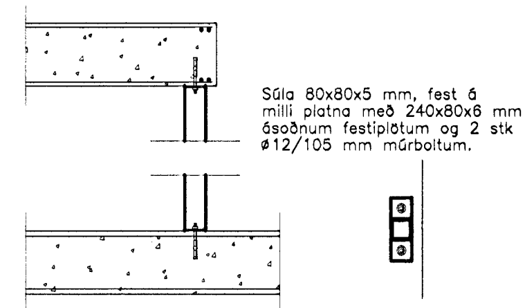
S2.7. Sála S2.7. 1:20. 8 | 9
