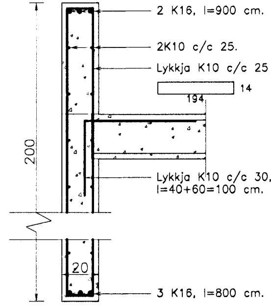
B2.1. Bíti B2.1. 1:20. 8 | 9
