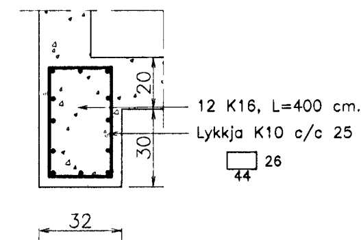
S2.1. Sála S2.1. 1:20. 8 | 9
