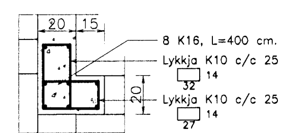
S2.4. Sála S2.4. 1:20. 8 | 9
