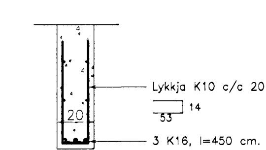
B1.5. Biti B1.5. 1:20.
