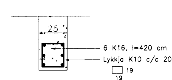
S1.5. Sála S1.5. 1:20.
