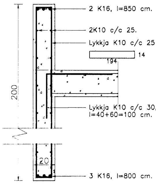
B1.1. Biti B1.1. 1:20.
