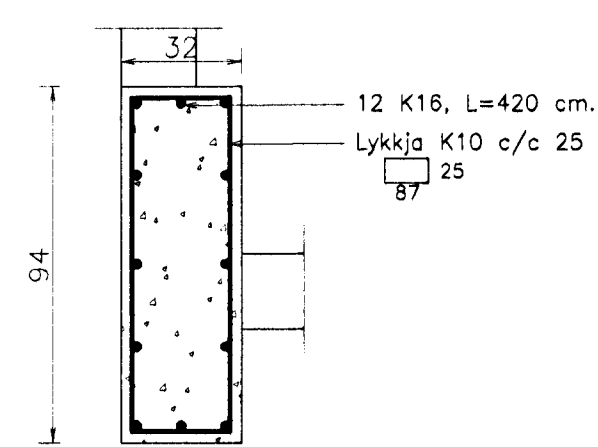
S1.7. Sála S1.7. 1:20.
