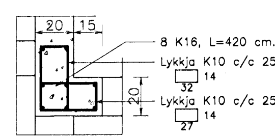
S1.5. Sála S1.5. 1:20.
