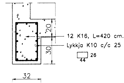
S1.1. Ógla S1.1. 1:20.
