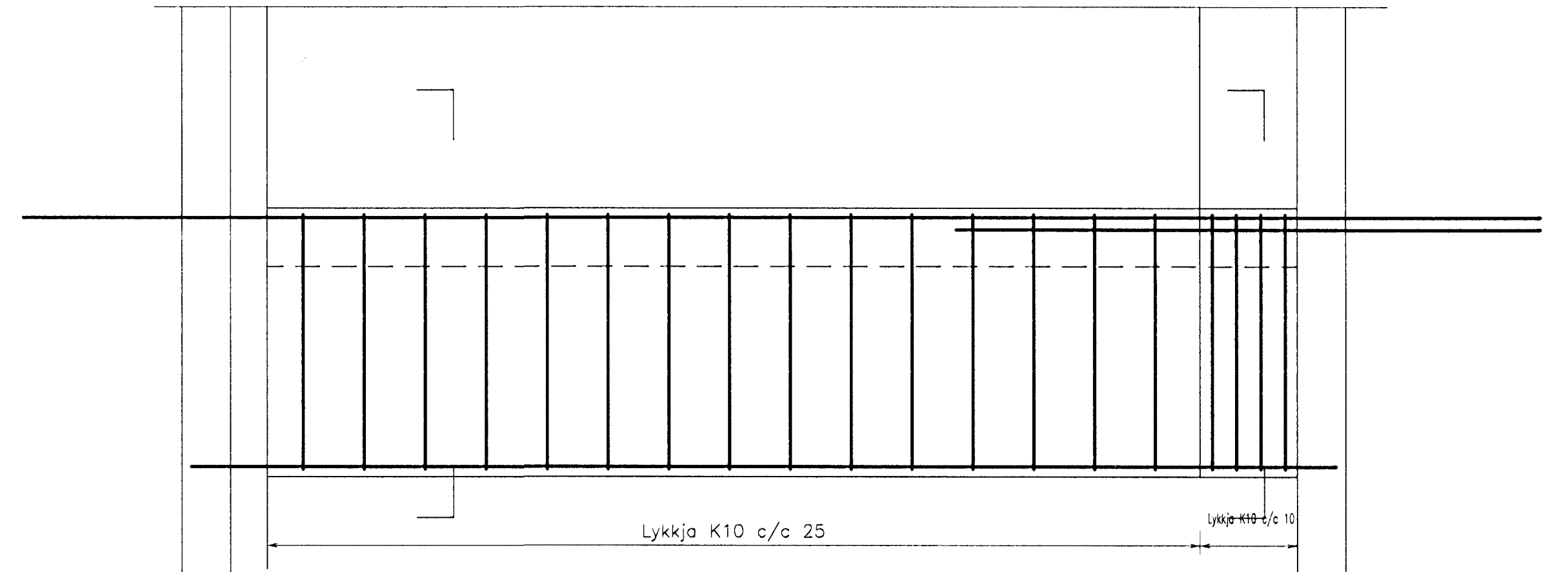
B1.4. Hliðarmynd og snið í biti B1.4. 1:20.
