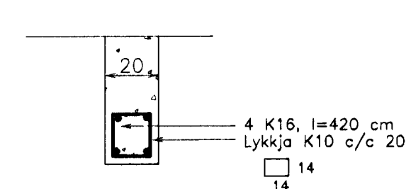
S1.6. Sála S1.6. 1:20.
