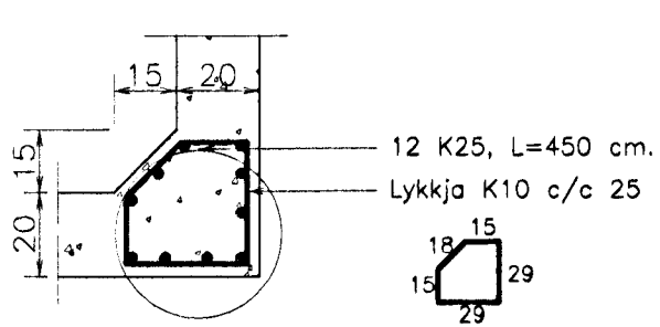
S1.8. Sála S1.8. 1:20.
