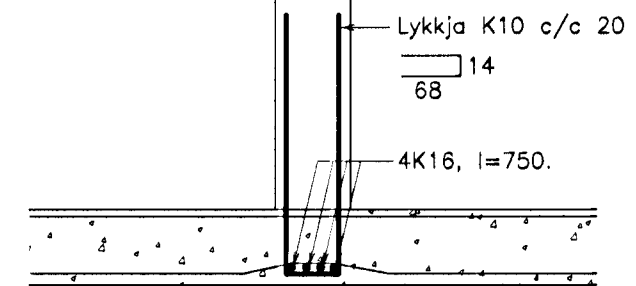
B0.2. Biti B0.2. 1:20.
