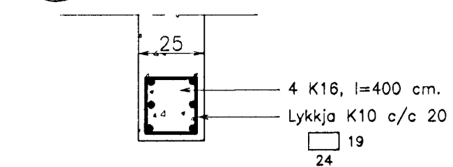
S0.6. Sála S0.6. 1:20.
