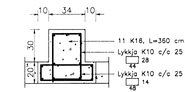
S0.2. Sála S0.2. 1:20.
