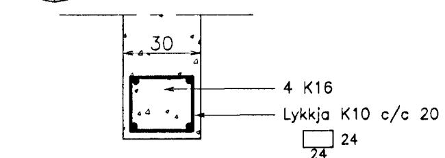
S0.4. Sála S0.4. 1:20.
