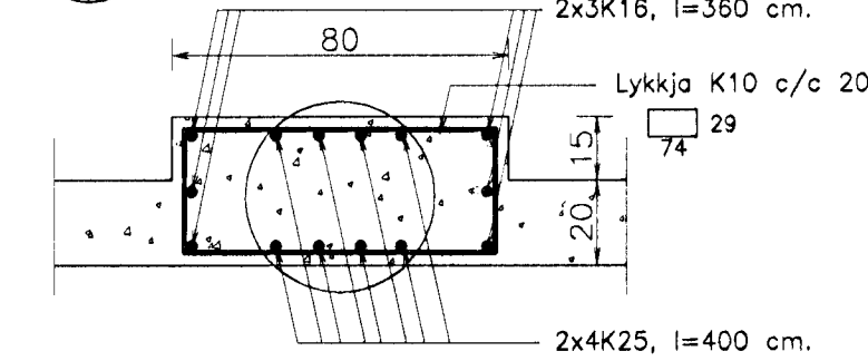
S0.5. Sála S0.5. 1:20.
