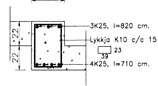
B0.1. Biti B0.1. 1:20.
