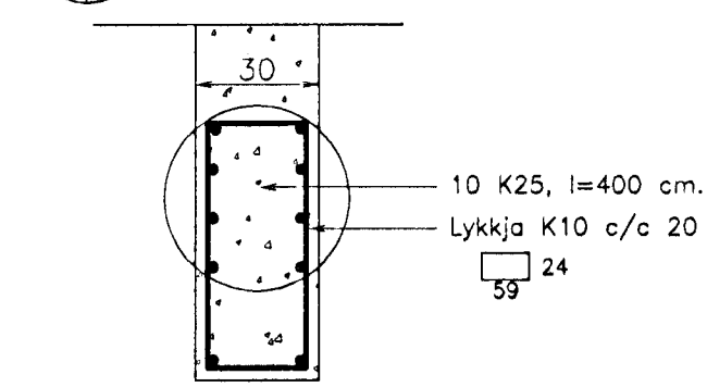
S0.3. Sála S0.3. 1:20.
