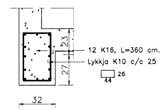
S0.1. Sála S0.1. 1:20.
