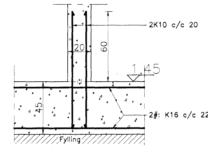
C Snið C-C. 1:20.
