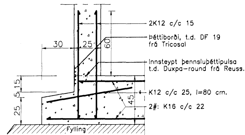
B Snið B-B. 1:20.
