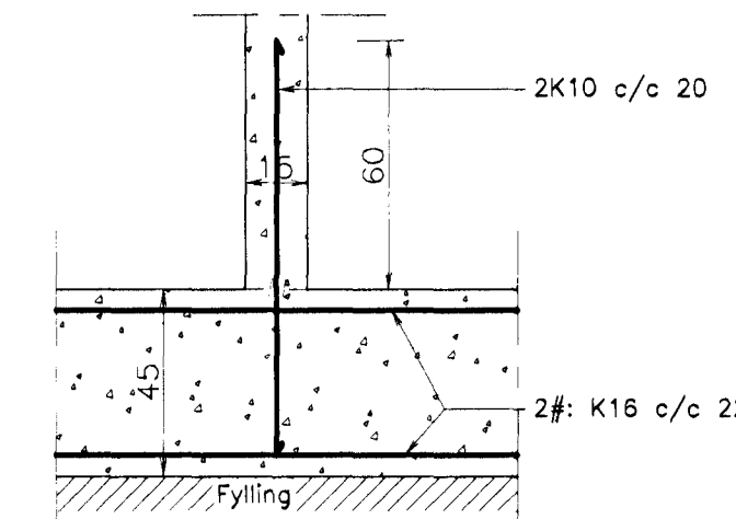
D Snið D-D. 1:20.
