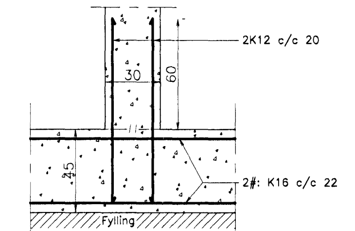
E Snið E-E. 1:20.
