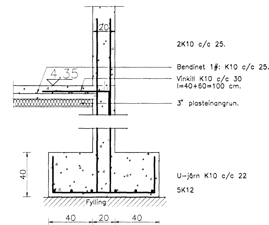
G Snið G-G. 1:20.
