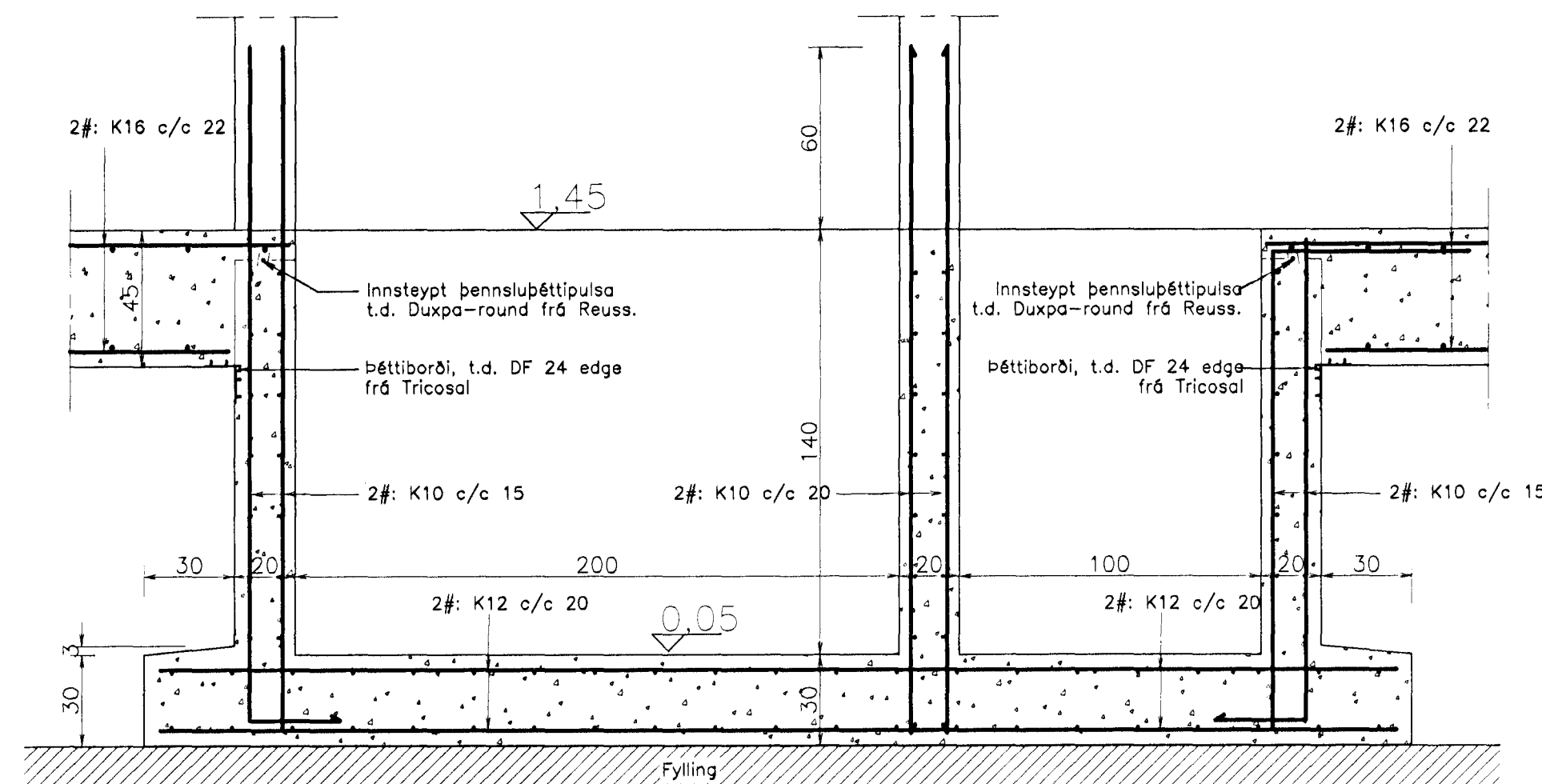
F Snið F-F. 1:20.
