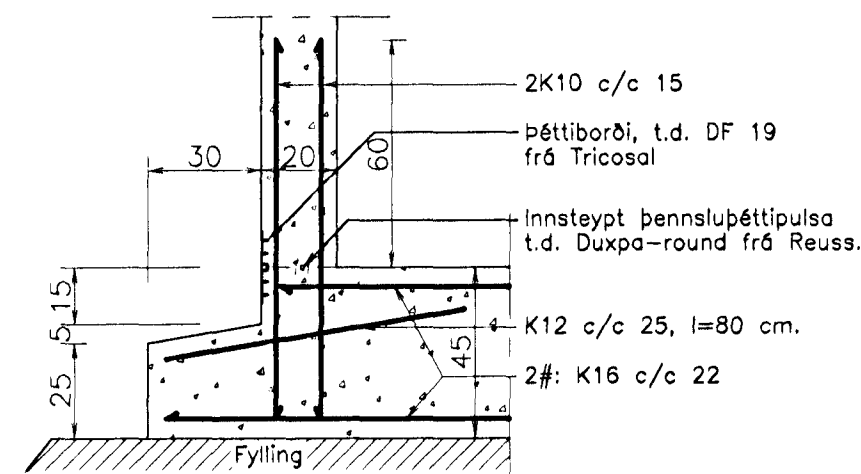
A Snið A-A. 1:20.
