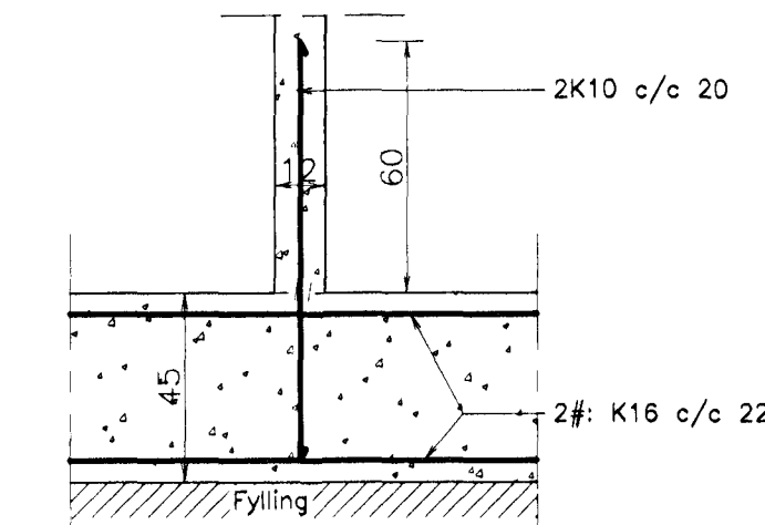
D Snið D-D. 1:20.
