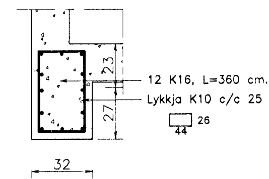
S0.1. Sála S0.1. 1:20.
