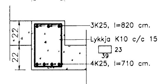
B0.1. Biti B0.1. 1:20.
