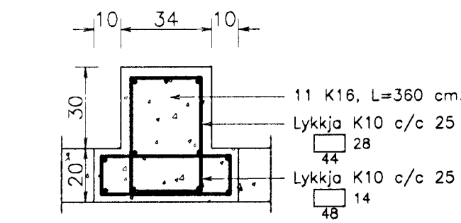
S0.2. Sála S0.2. 1:20.
