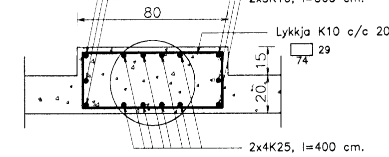
S0.5. Sála S0.5. 1:20.
