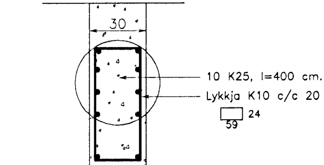
S0.3. Sála S0.3. 1:20.
