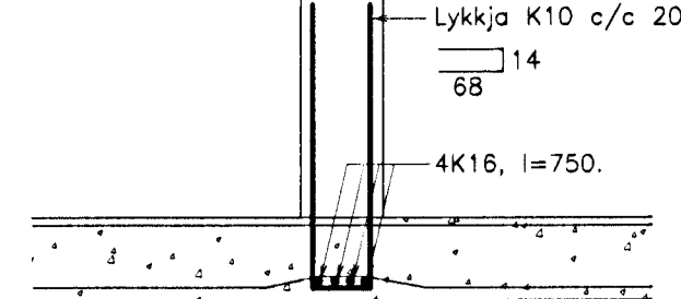
B0.2. Biti B0.2. 1:20.
