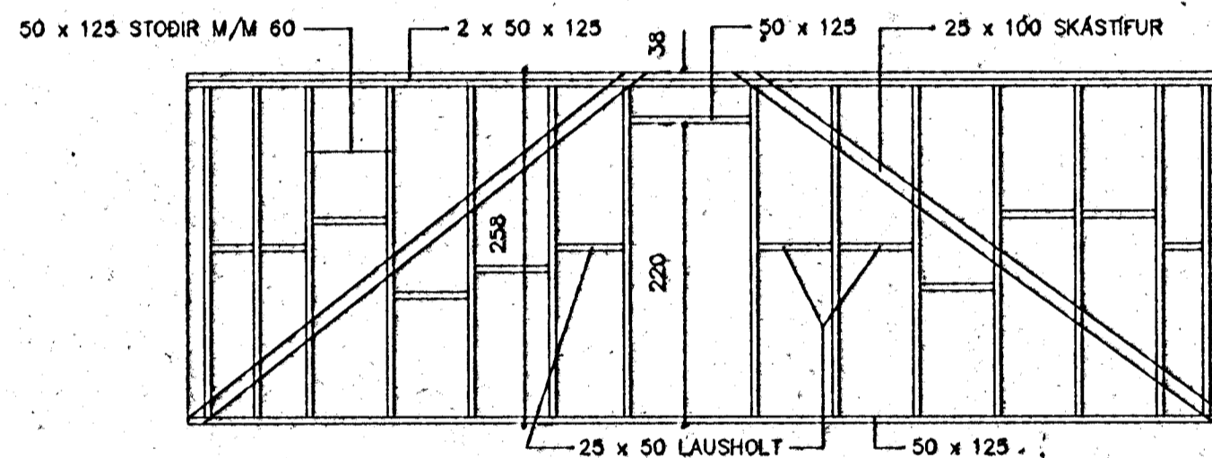
AUSTURHLIÐ, M=1:50
