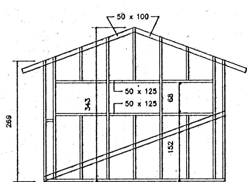
NORÐURHLIÐ, M=1:50
