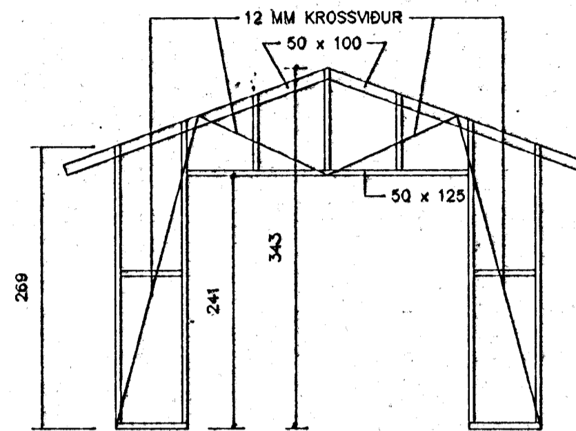
SUÐURHLIÐ, M=1:50
