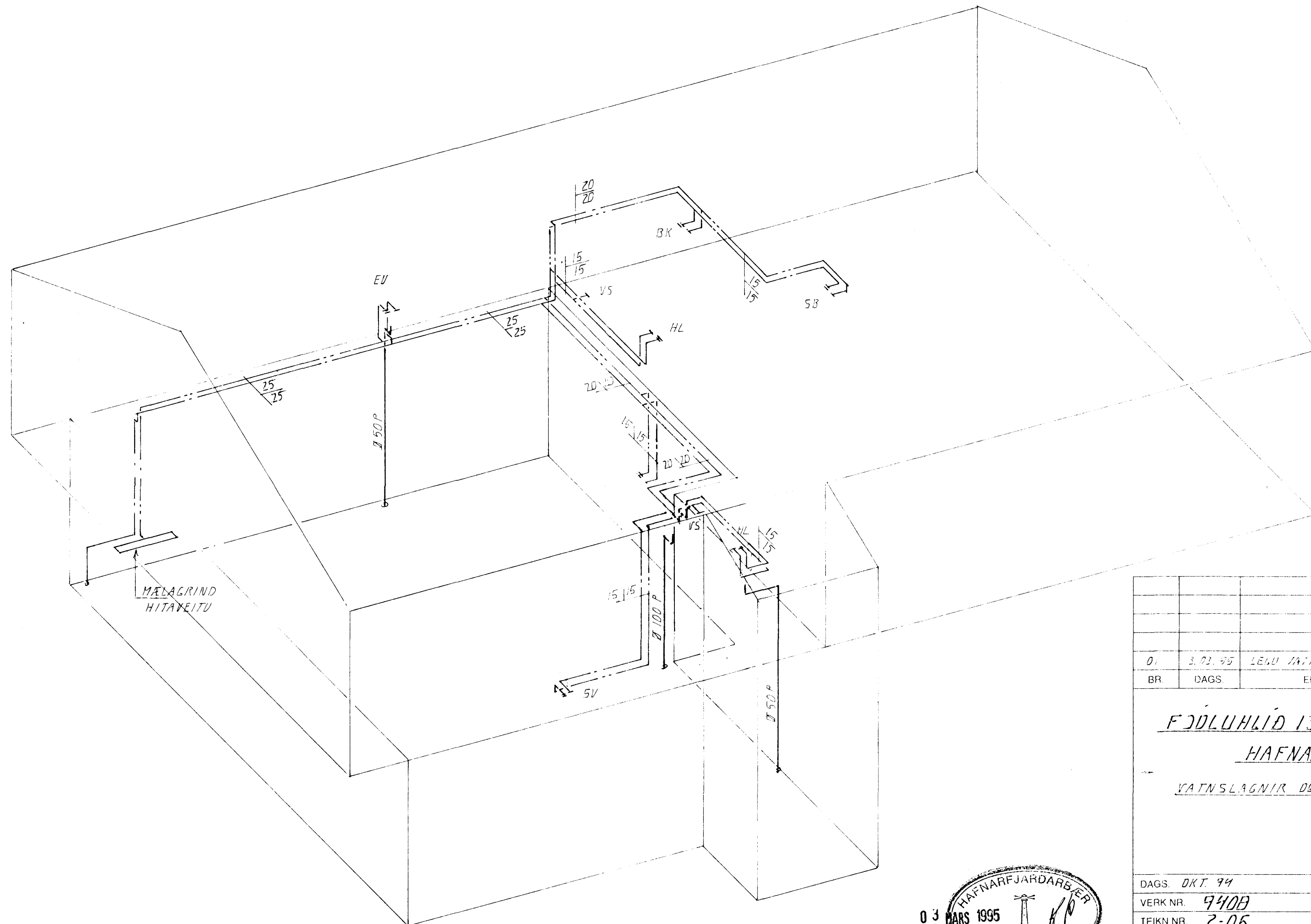
RÚMMYND VATNSLAGNA. 1:50
