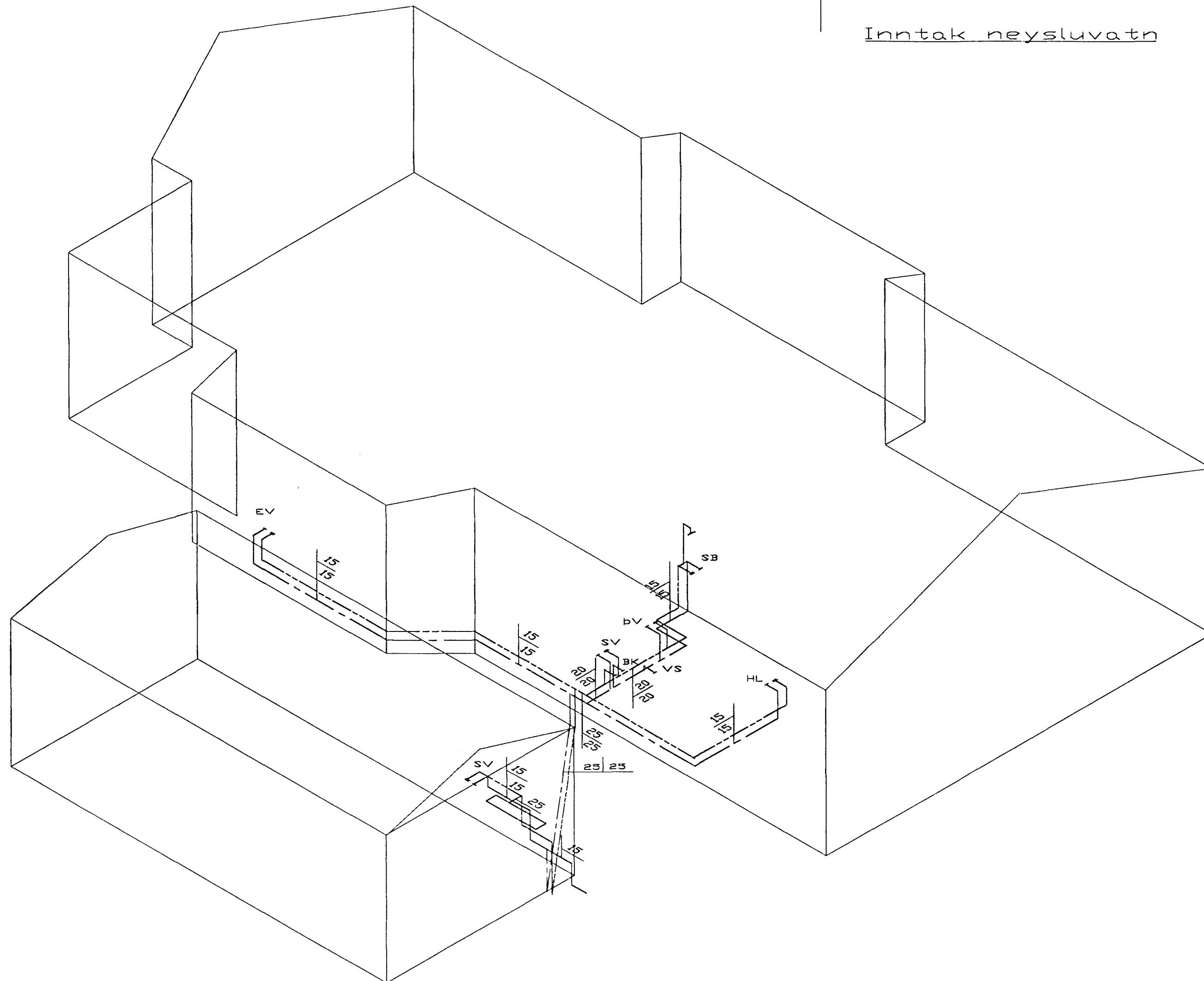
RÚMMYND - VATNSLAGNA 1:50
